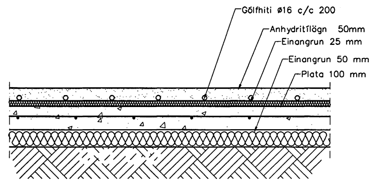
Hita- og Neysluvatnslagnir, Snið í botnplötu, 1:10
