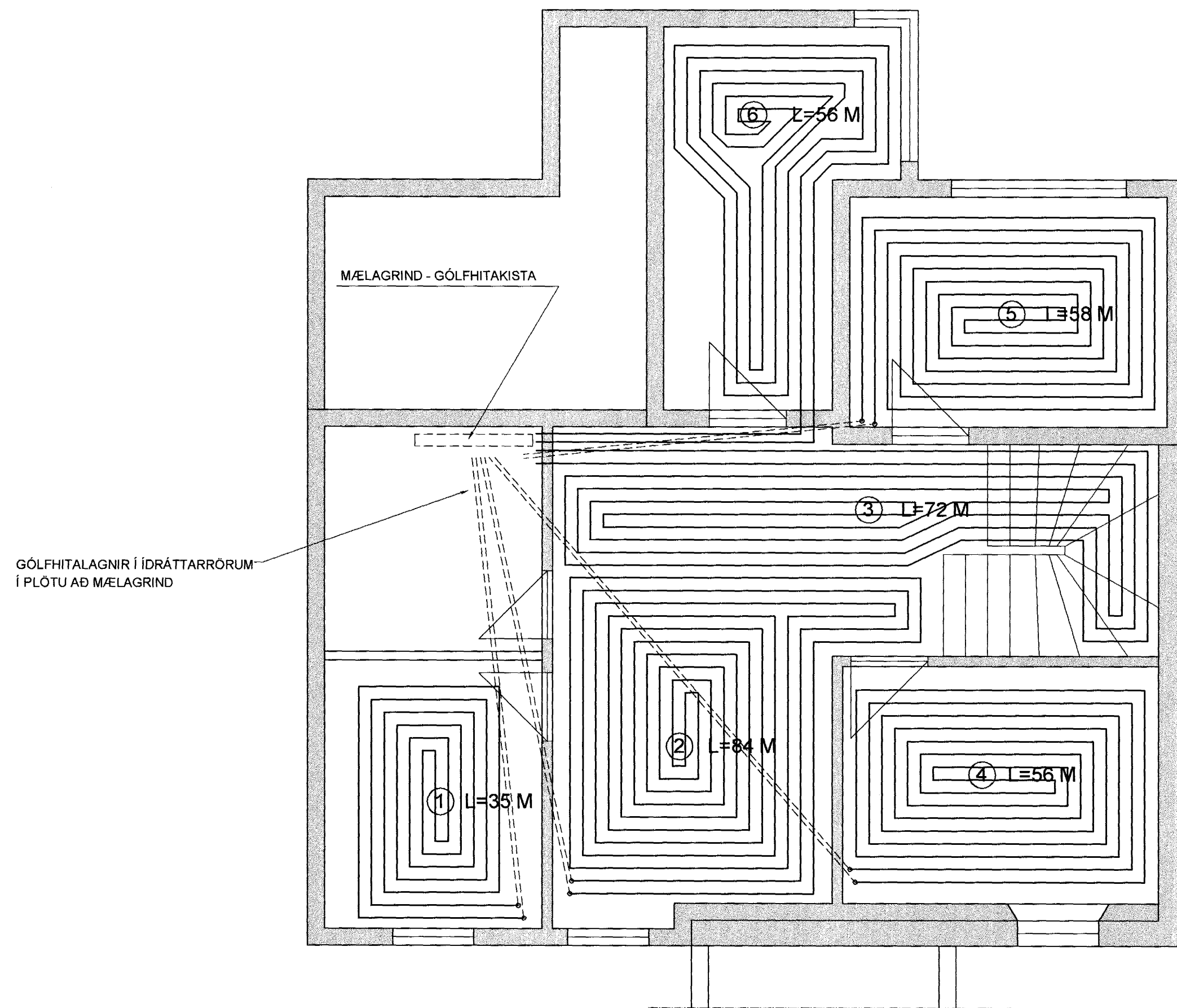
GRUNNMYND NEDRI HÆÐAR 1:50
