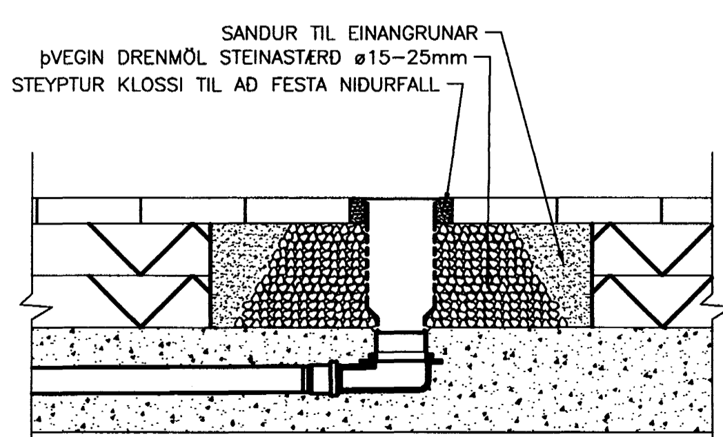
B SNID þar sem engin einangrun er 4001 1:10
