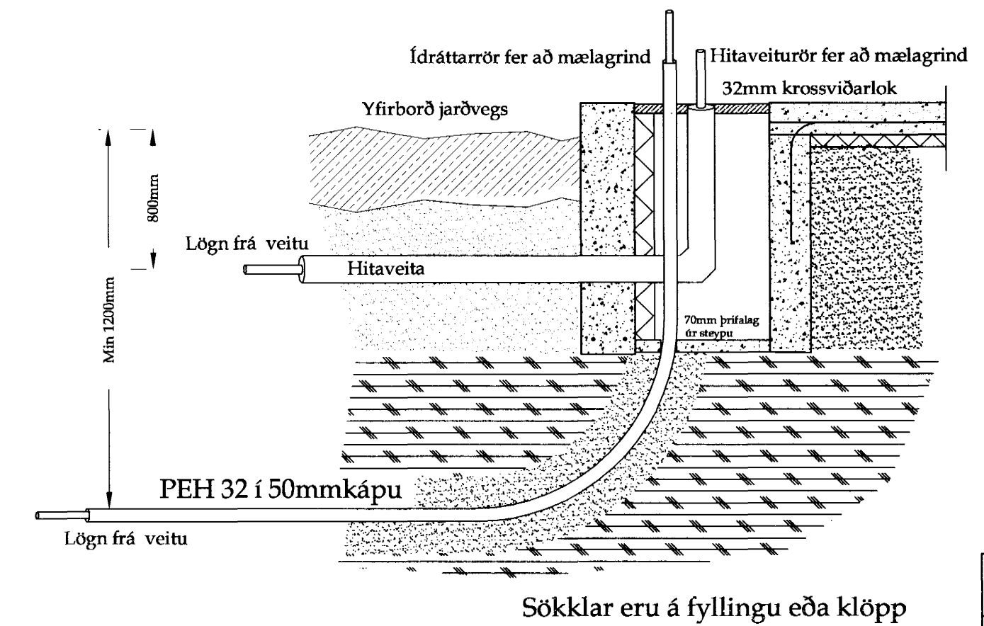
01 Snið 01 1-02 Mk. 1:20
