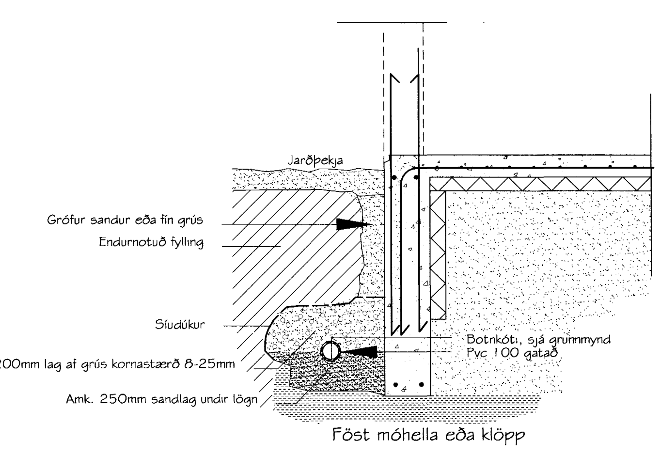
Snið í frágang á drenlagn
