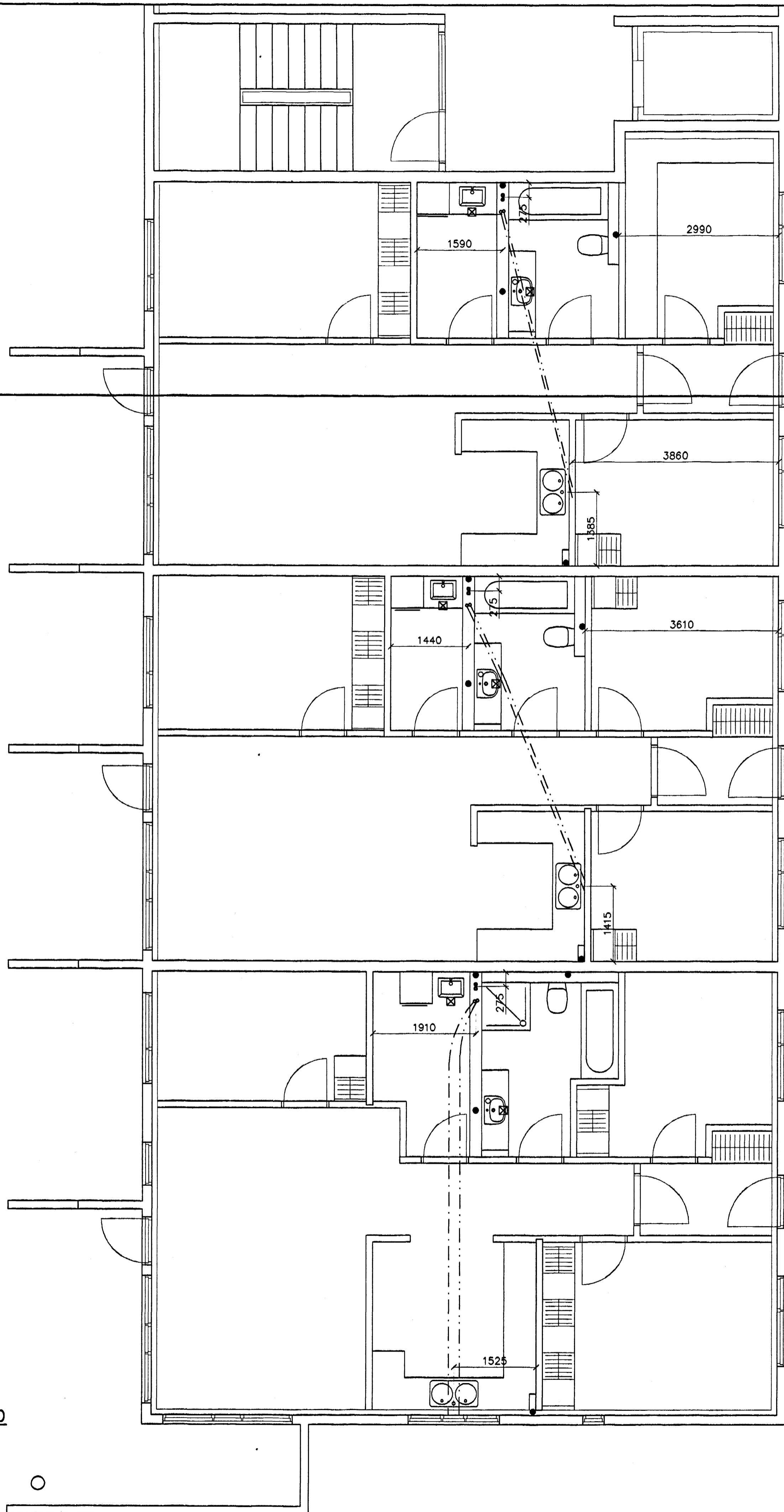
GRUNNMYND 1 HÆÐAR 1:50
