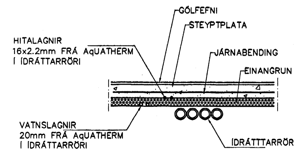
LAGNIR, SNIÐ, 1:20
