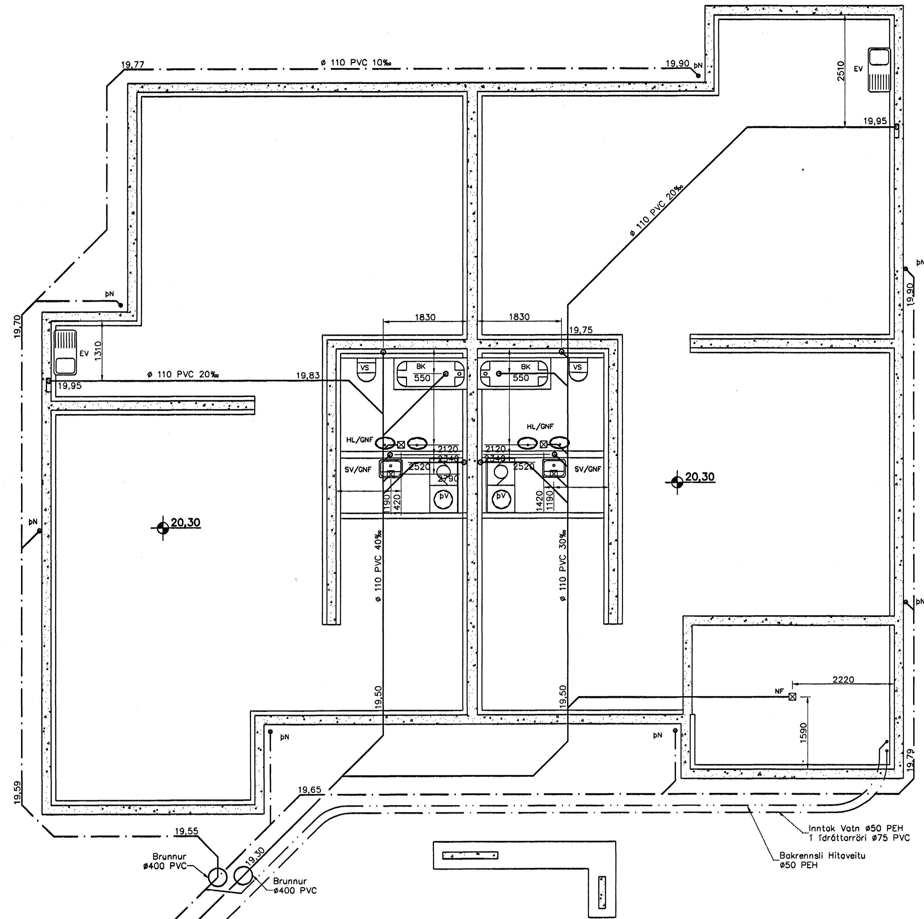
Grunnlagnir. Grunnmynd. 1:50
