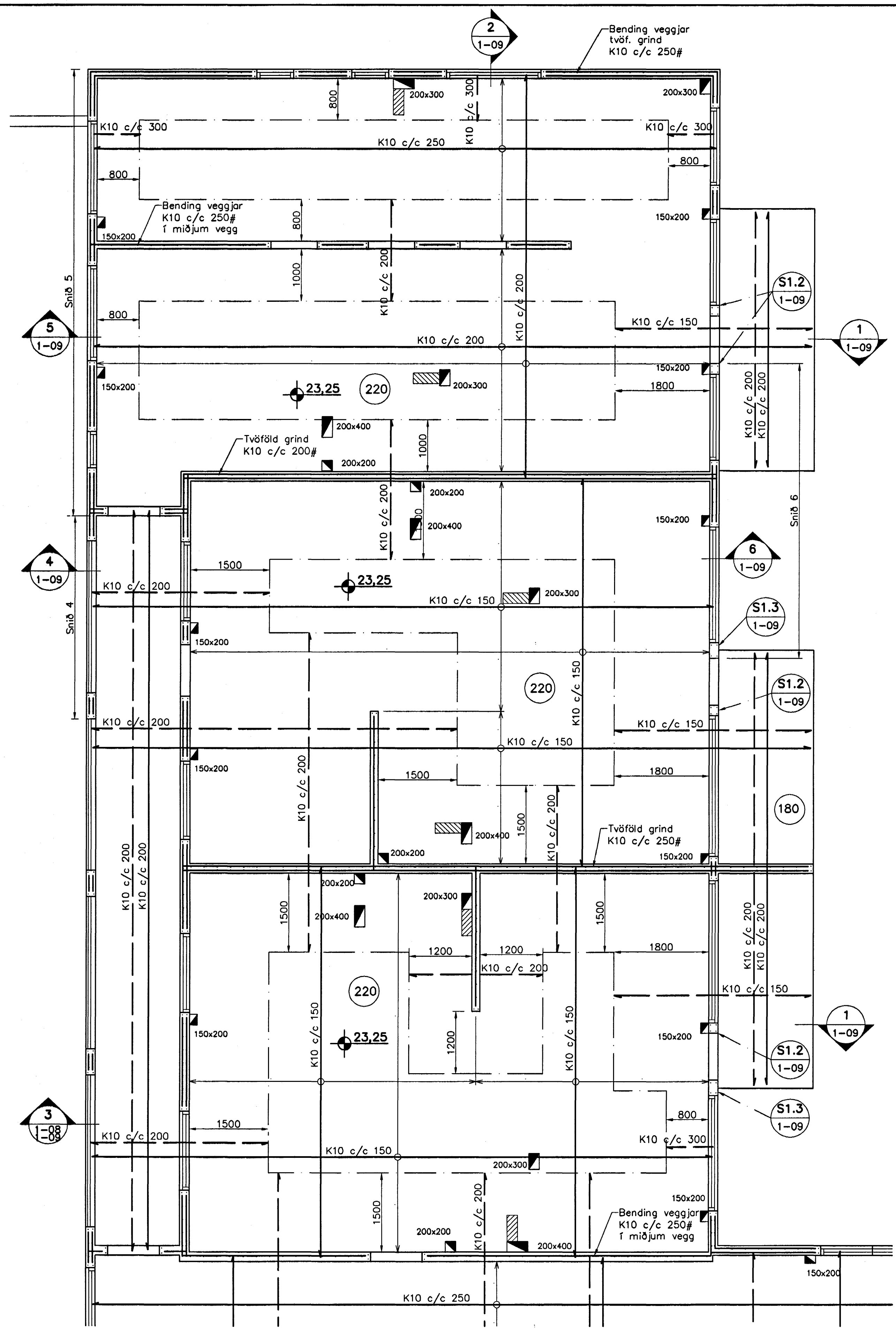
Veggir 2. hæð, Plata yfir 2. hæð, Grunnmynd, 1:50
