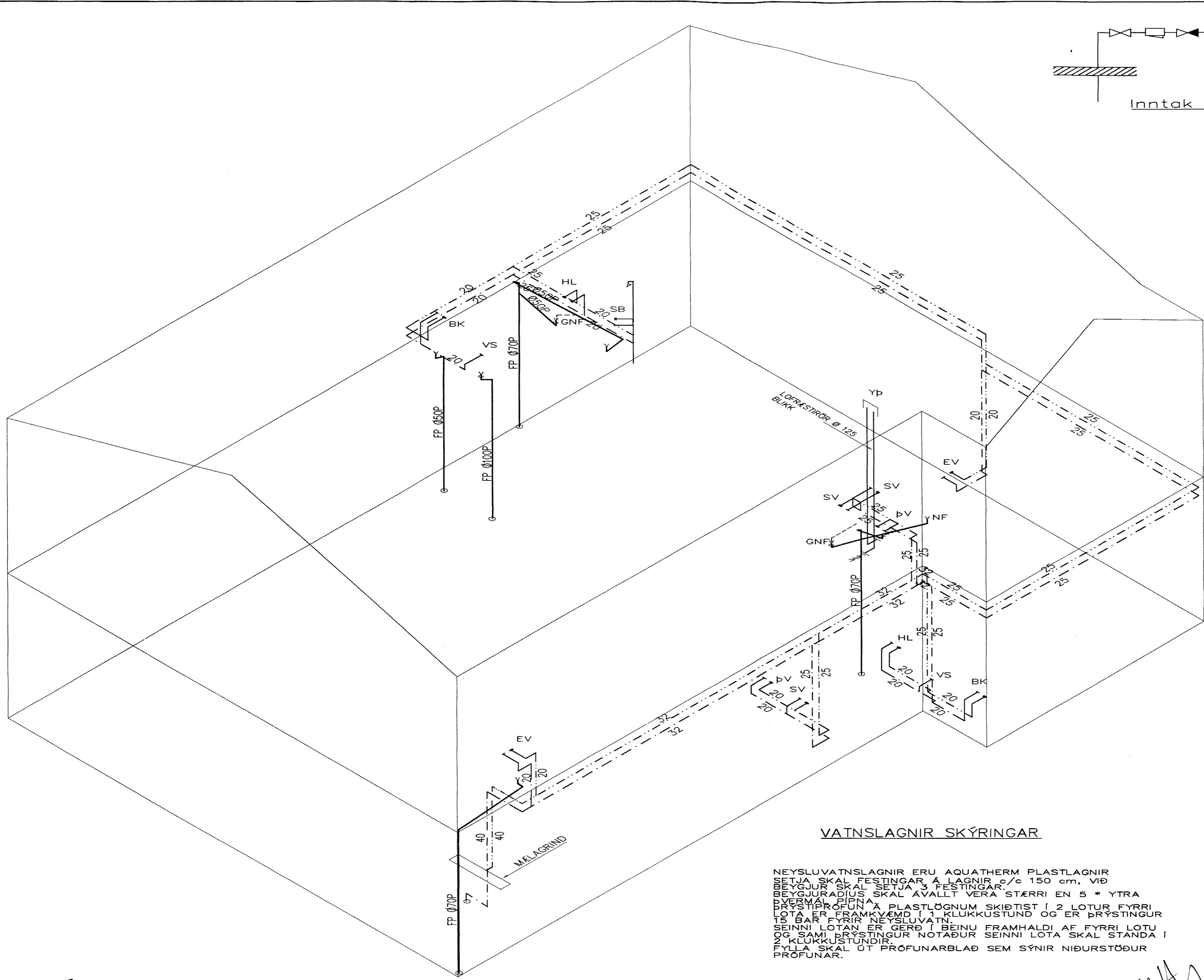
RÚMMYND VATNSLAGNA 1:50
