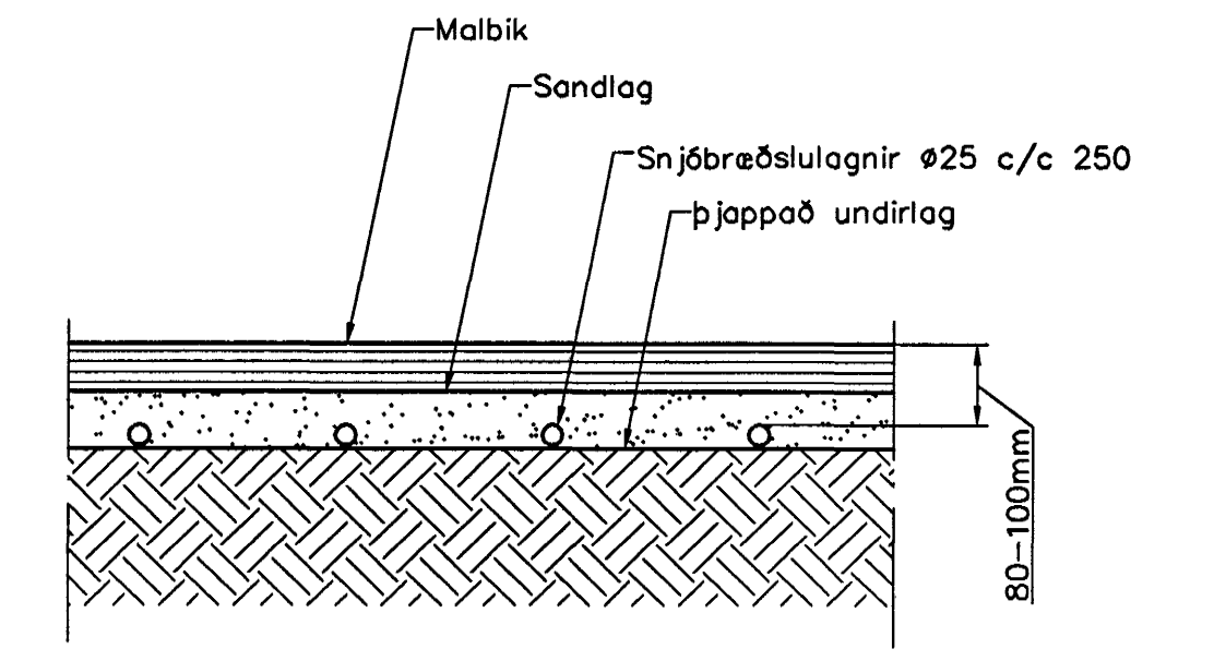
Snjóbræðslulagnir, Snið, 1:10
