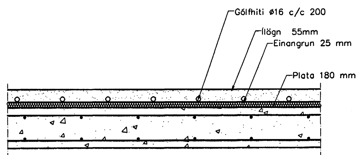
Gólfhiti, Snið 1 milliþötu, 1:10
