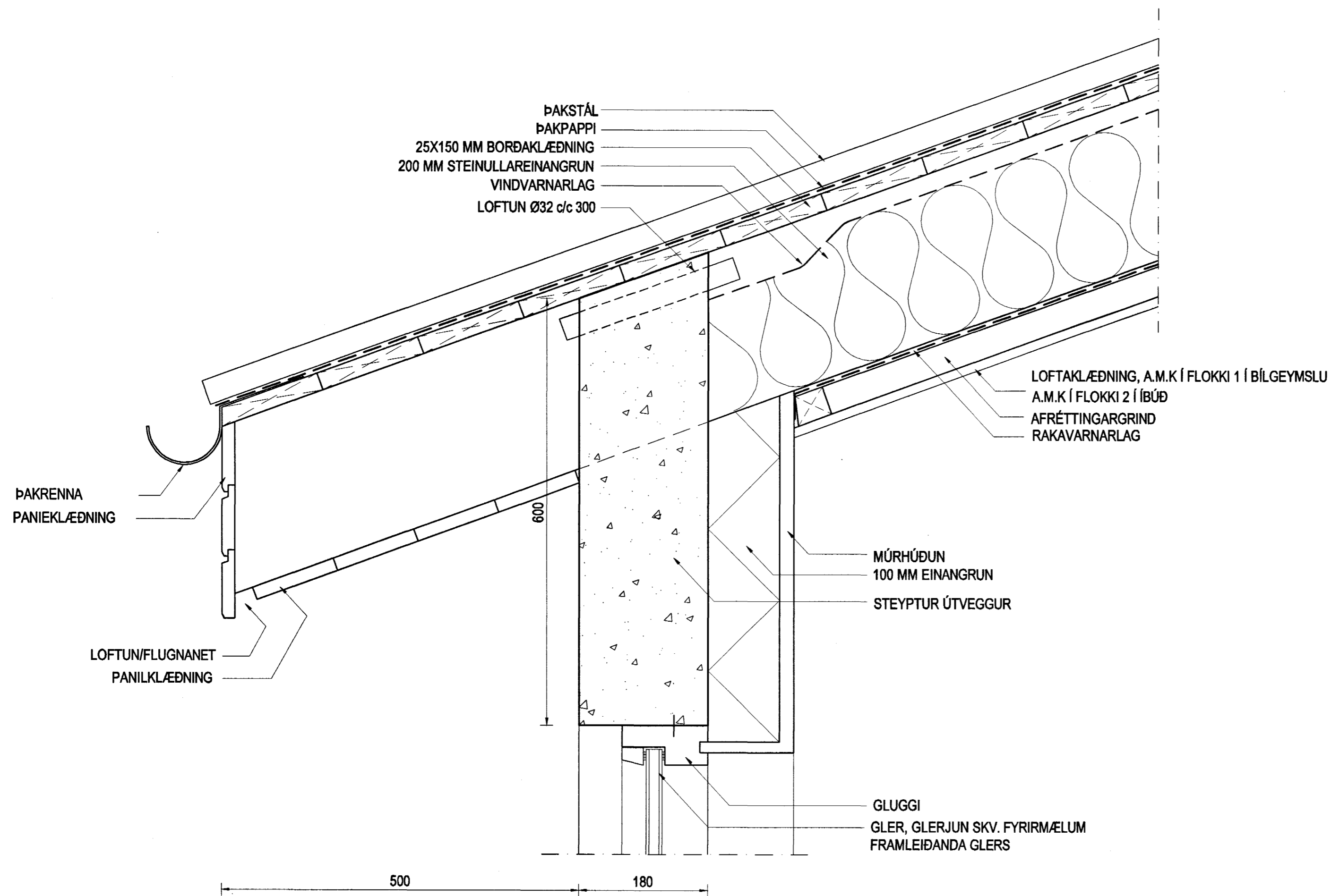
ÞAKBRÚN MKV. 1:5
