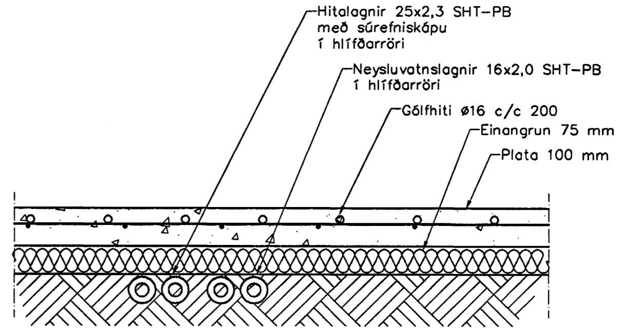
Hita- og Neysluvatnslagnir, Snið í botnplötu, 1:10
