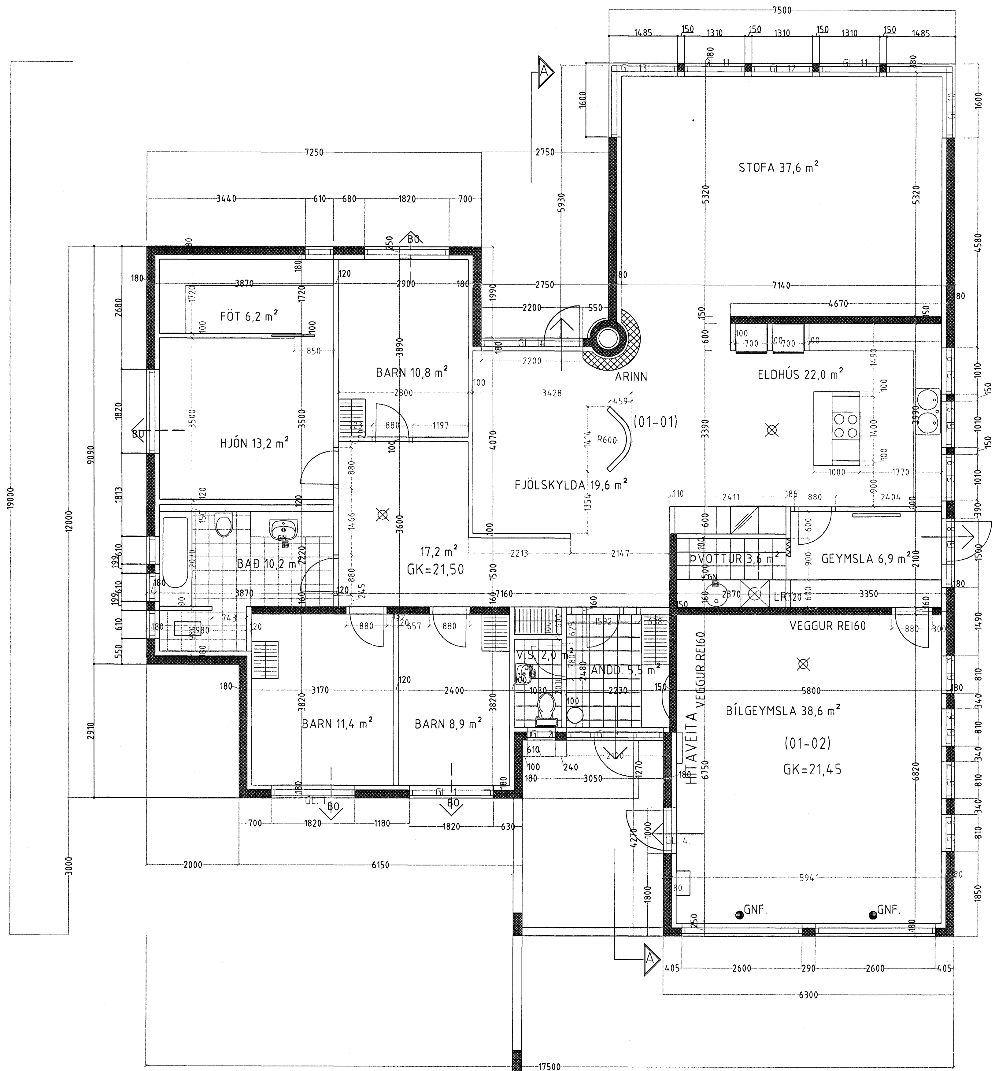
GRUNNMYND MKV. 1:50.
