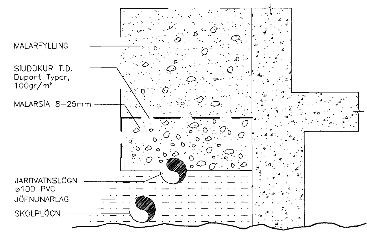
FRÁGANGUR JARÐVATNSLAGNA ÚR PVC 1:10
