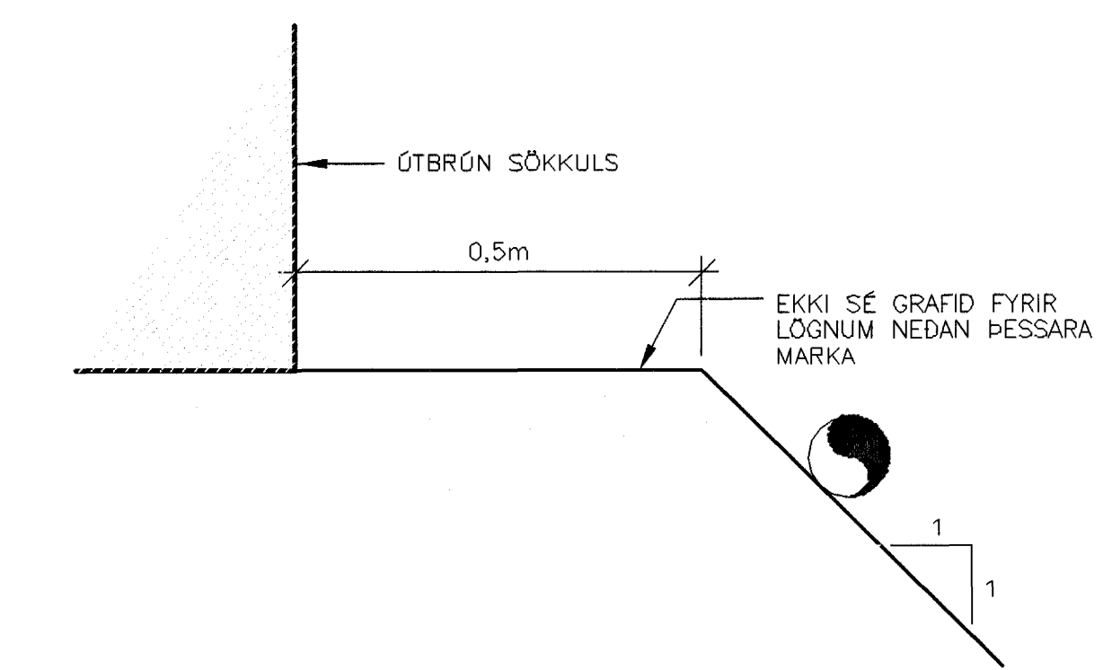
LEGA LAGNA VÍÐ HÚS 1:10
