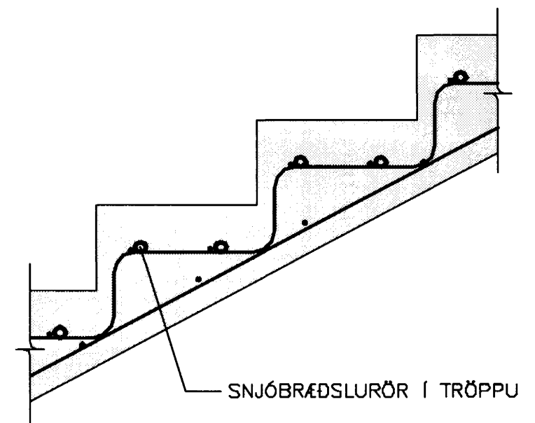
SNID Í SNJÓBRÆDSLULÖGN Í STEYPTUM TRÖPPUM
