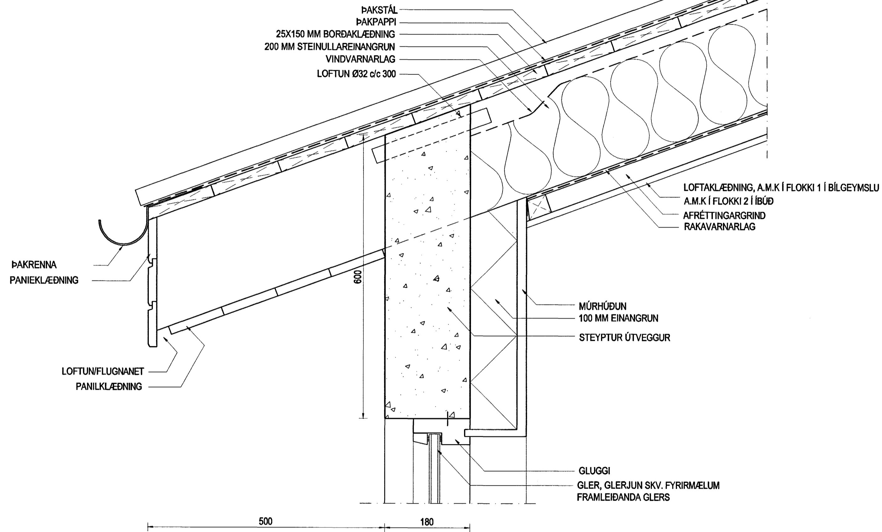
ÞAKBRÚN MKV. 1:5
