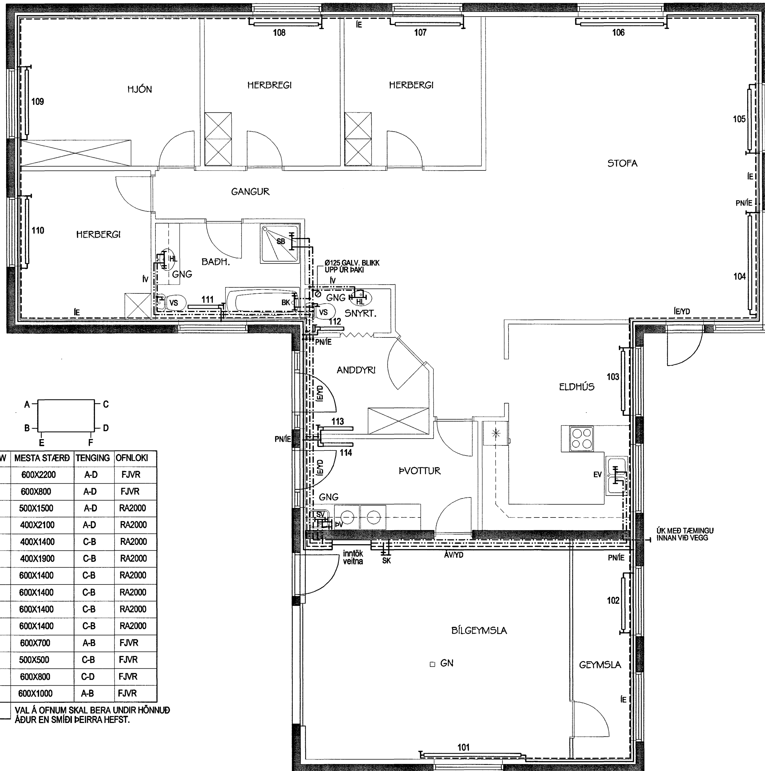
NEYSLUVATNS- OG HITLAGNIR, GRUNNMYND MKV. 1:50
