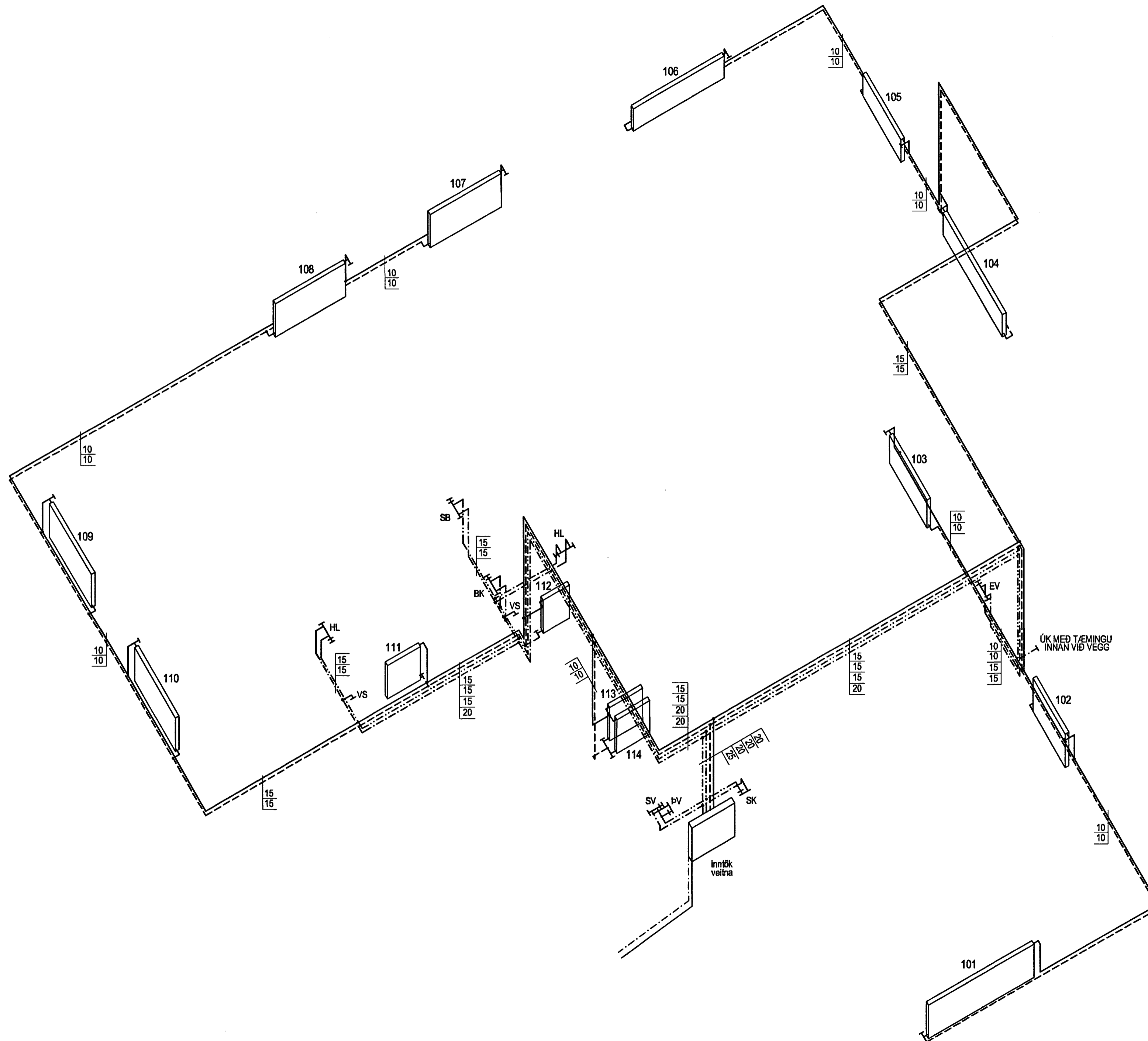
NEYSLUVATNS- OG HITALAGNIR, RÚMMYND MKV. 1:50
