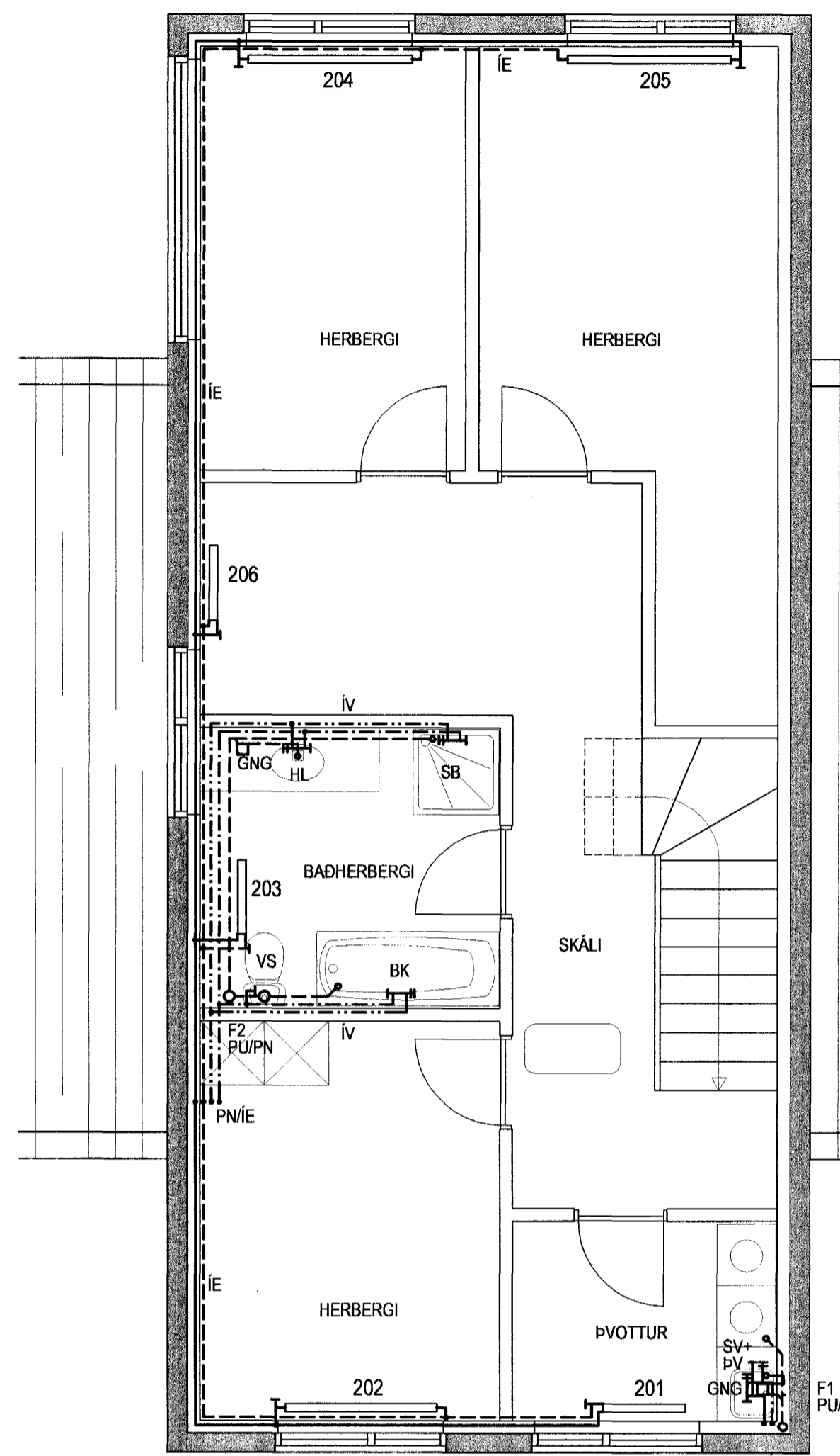
FÍFUVELLIR 19 NEYSLUVATNS- OG HITLAGNIR GRUNNMYND EFRÍ HÆÐAR MKV. 1:50
