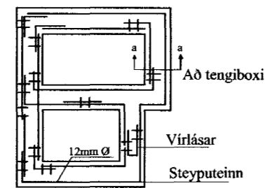
Grunnmynd sökkulvegja
