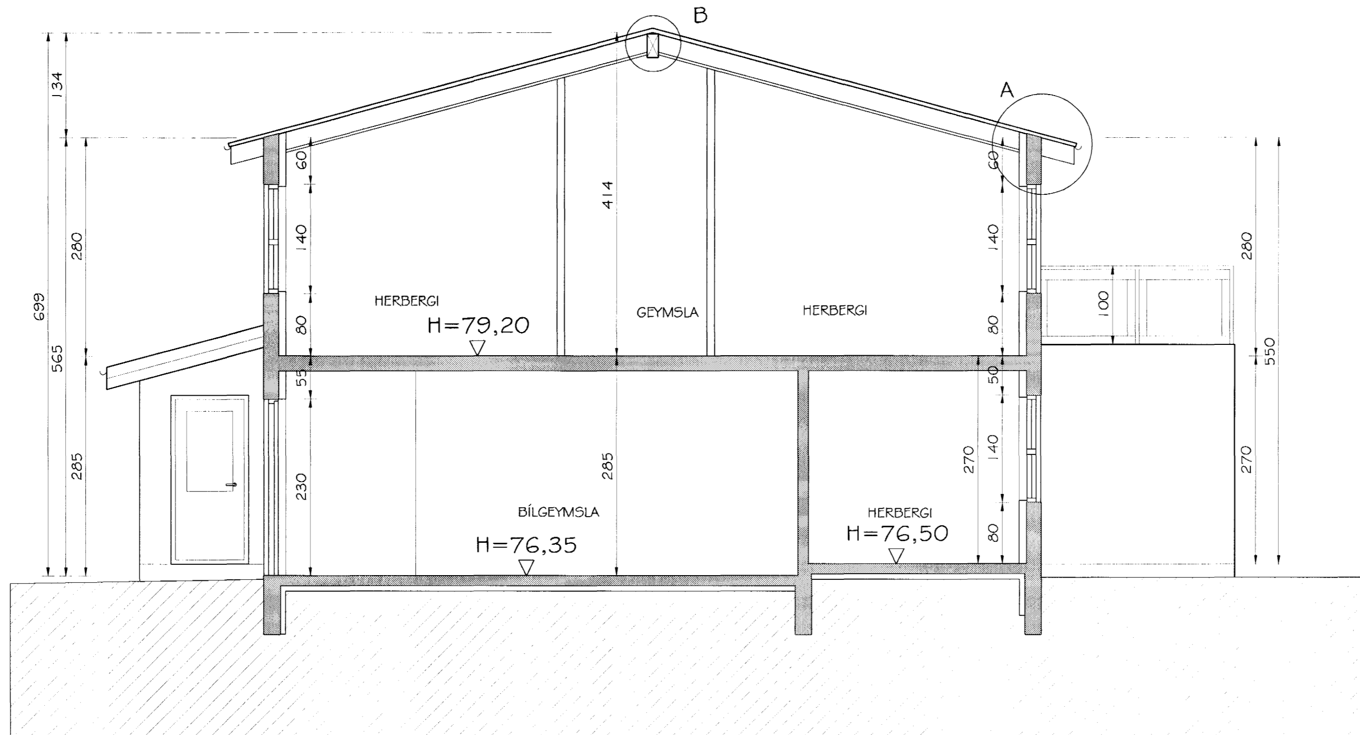
SVÖLUÁS 5 SNIÐ A-A MKV. 1:50
