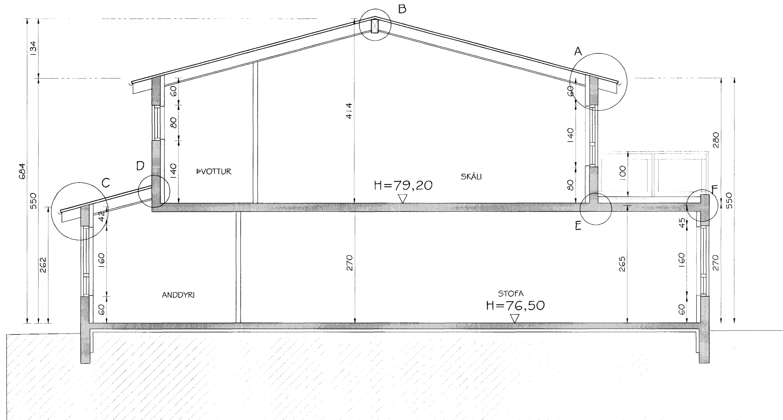
SVÖLUÁS 5 SNID B-B MKV. 1:50
