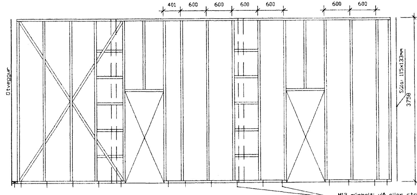
Grind 17 innveggur Nákvæm staðsetning innhurða, s.j.s sérteikningu aðalhönnuðar. M12 gárbolti við allar stöðir. Borðrými í steypu 80mm Skinnur 40x40x4
