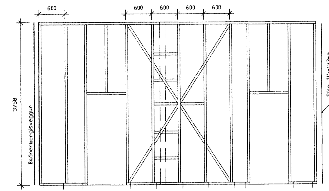
Grind 18 innveggur Nákvæm staðsetning innhurða, s.j.s sérteikningu aðalhönnuðar.
