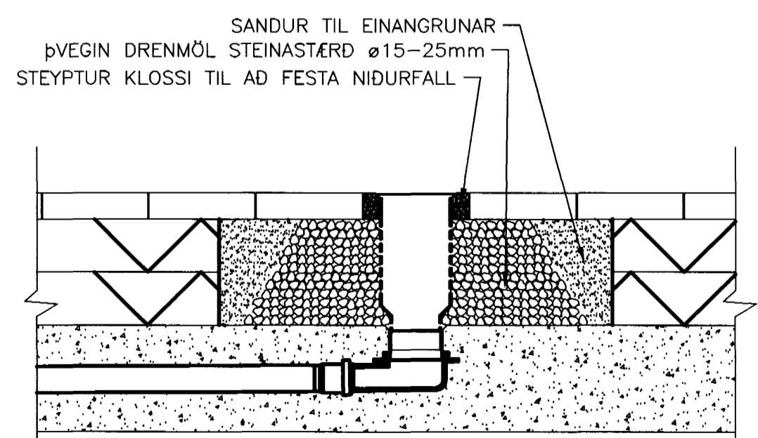
SANDUR TIL EINANGRUNAR ÞVEGIN DRENMÖL STEINASTÆRD ø15-25mm STEYPTUR KLOSSI TIL AD FESTA NIDURFALL B SNID þar sem engin einangrun er 4001 1:10
