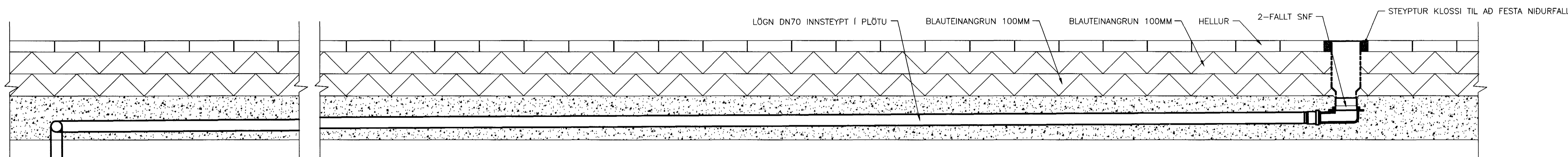
NIDURFALLSLÖGN Í EINANGRUN Á VEGG A SNID þar sem engin einangrun er 4001 1:10
