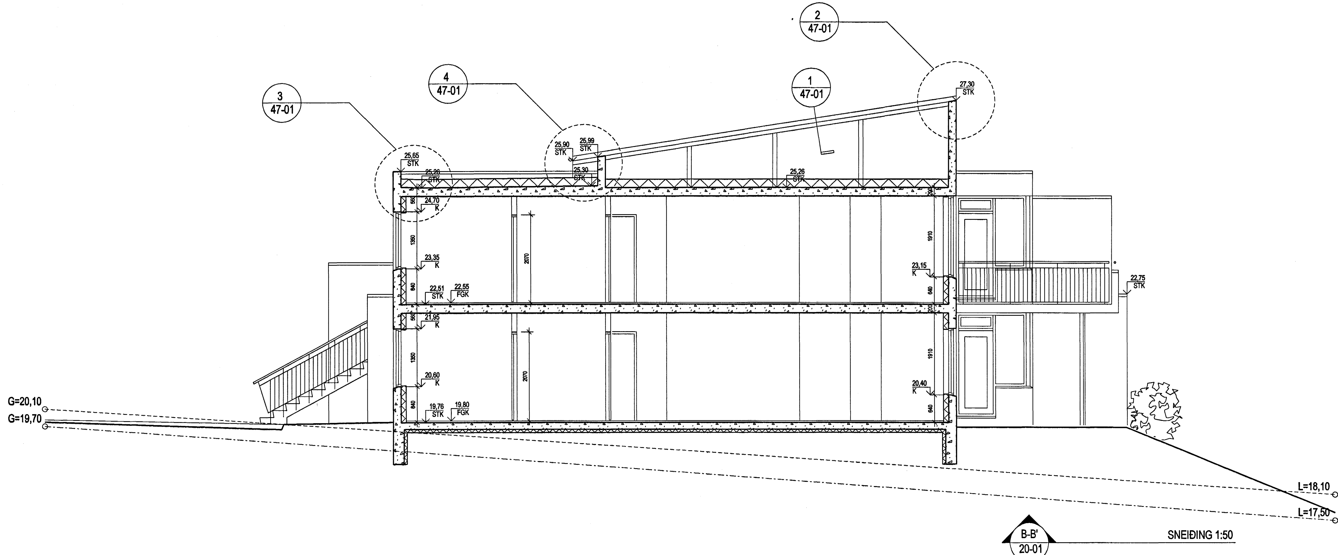
A-A' 20-01 SNEIDING 1:50
