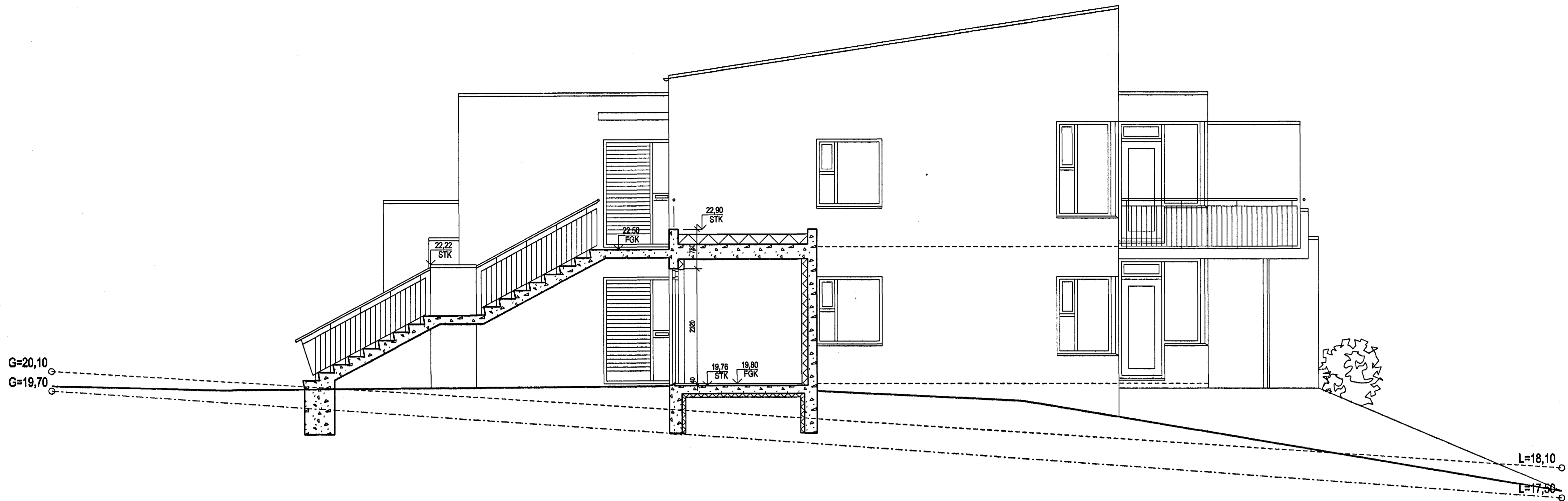
C-C' 20-01 SNEIÐING 1:50
