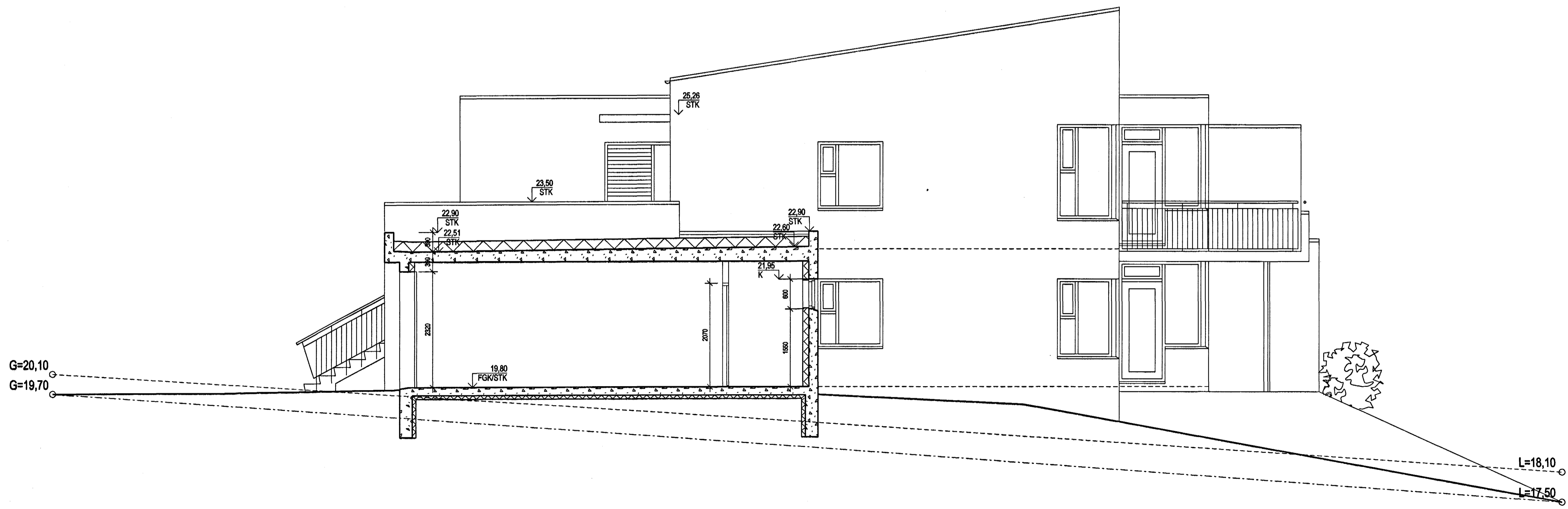
C-C' 20-01 SNEIÐING 1:50
