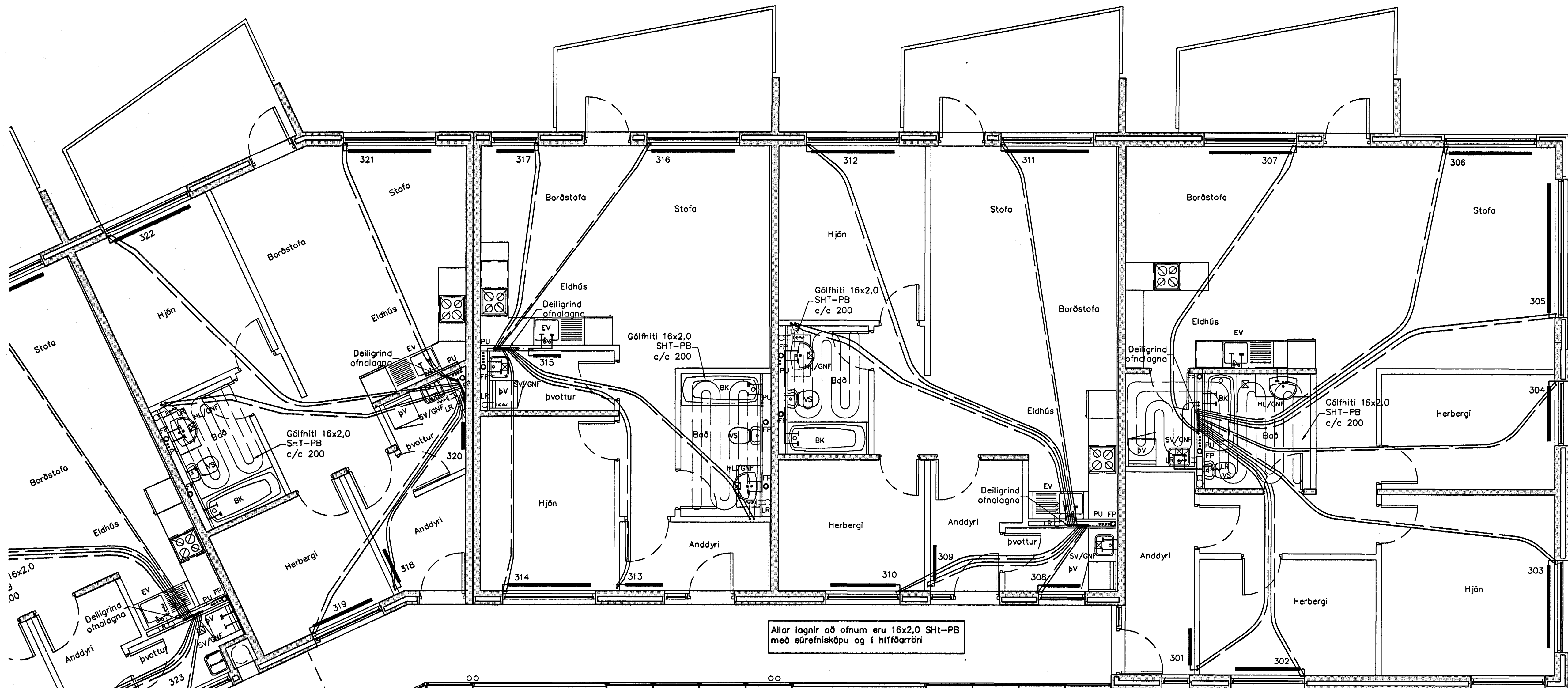
Lagnir 3. Hæð, Grunnmynd, 1:50
