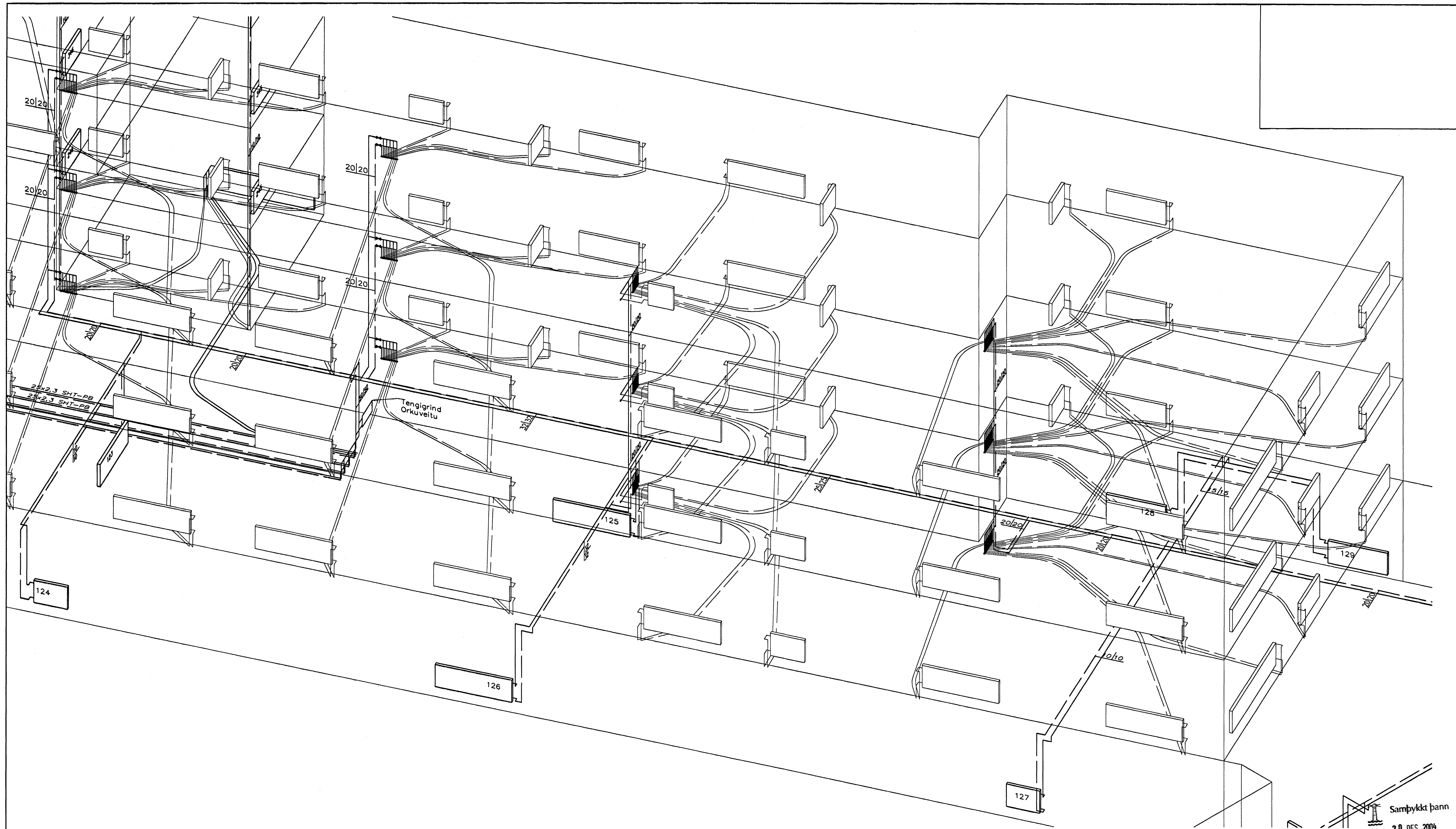
Hitalagnir, Rúmmynd, 1:50
