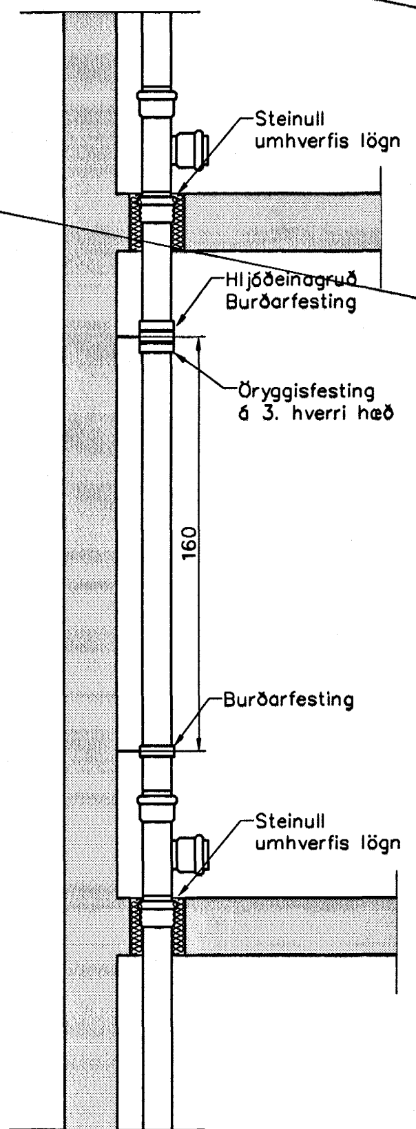
Fallpípa, festingar 1:20
