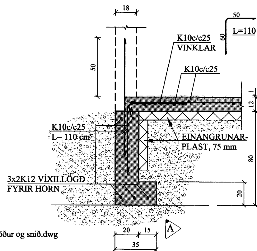
A2 SNIÐ. 1:20 1-02
