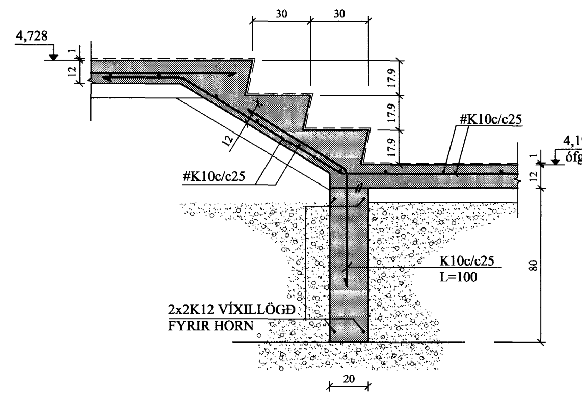
C2 SNIÐ. 1:20 1-02
