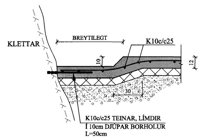
B2 SNIÐ. 1:20 1-02
