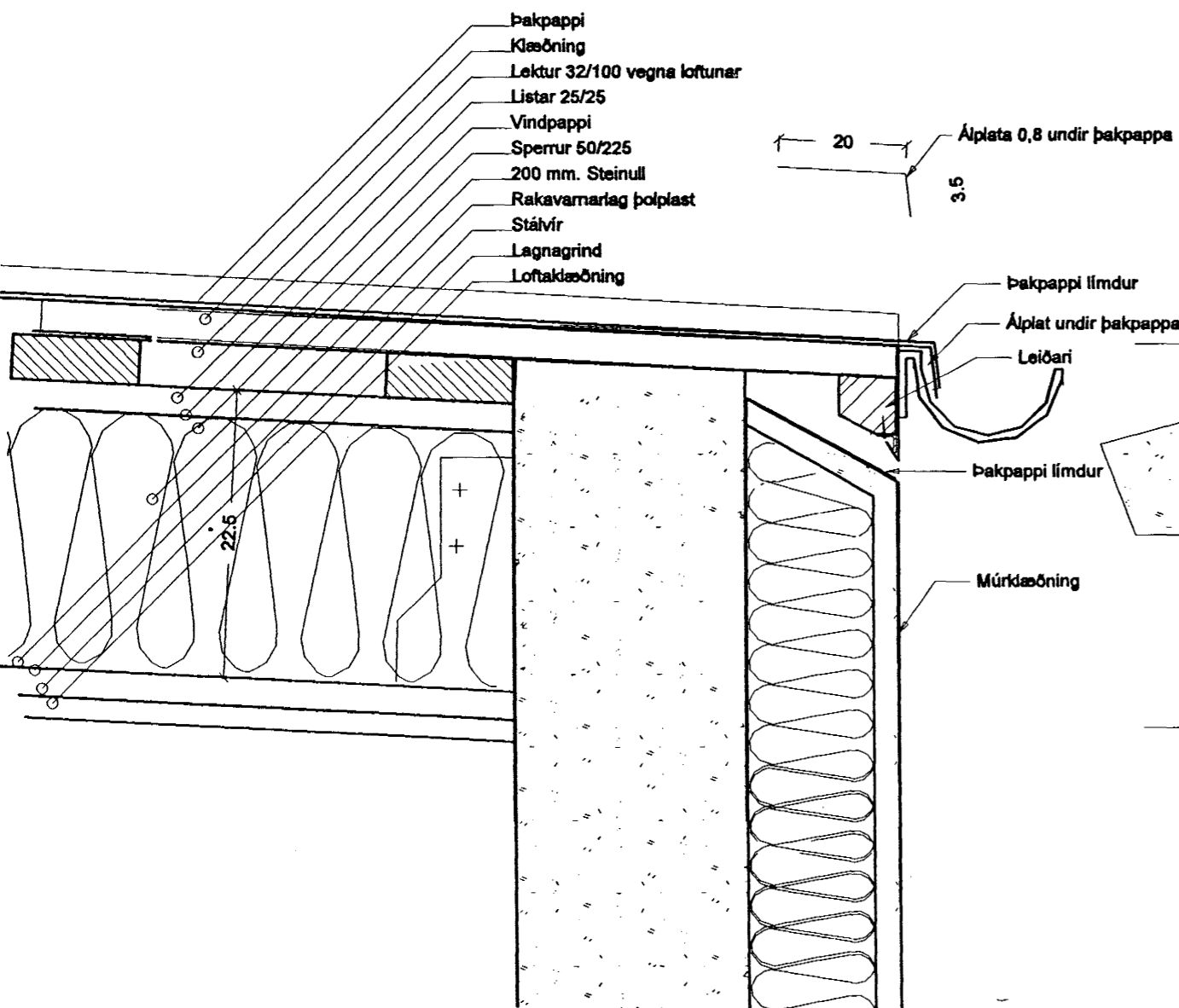
V-5. Lóðrétt snið í útvegg/þak.
