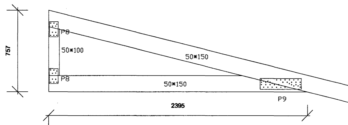
KRAFTSPERRA (D) MKV. 1:20 5 stk.
