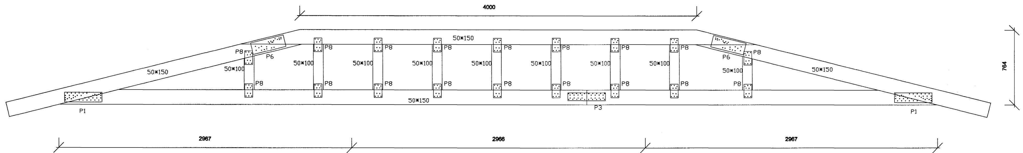
KRAFTSPERRA (C) MKV. 1:20 1 stk.
