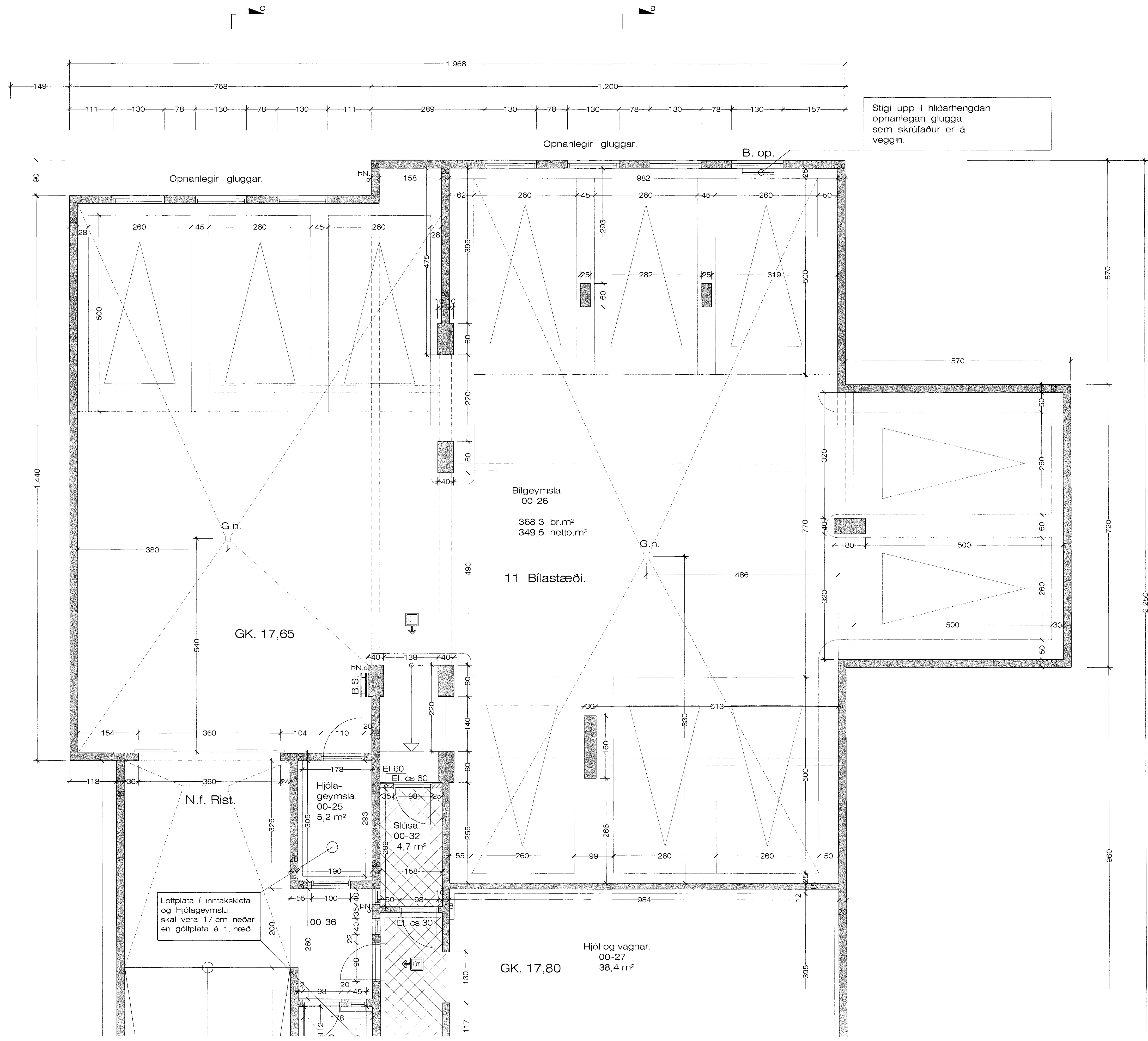
Grunnmynd. Kjallara. B 1:50
