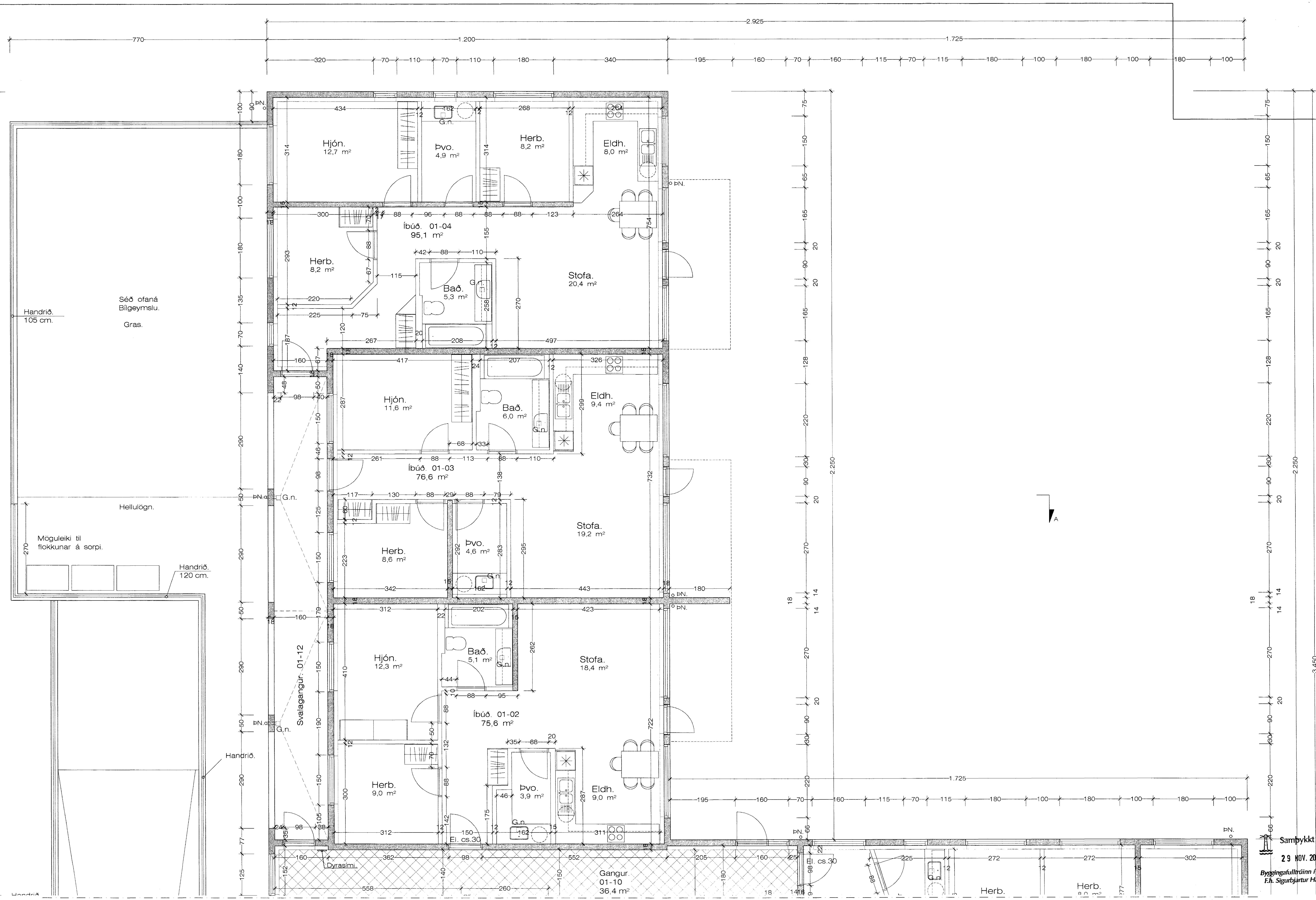
Grunnmynd. Jarðhæðar. B 1:50
