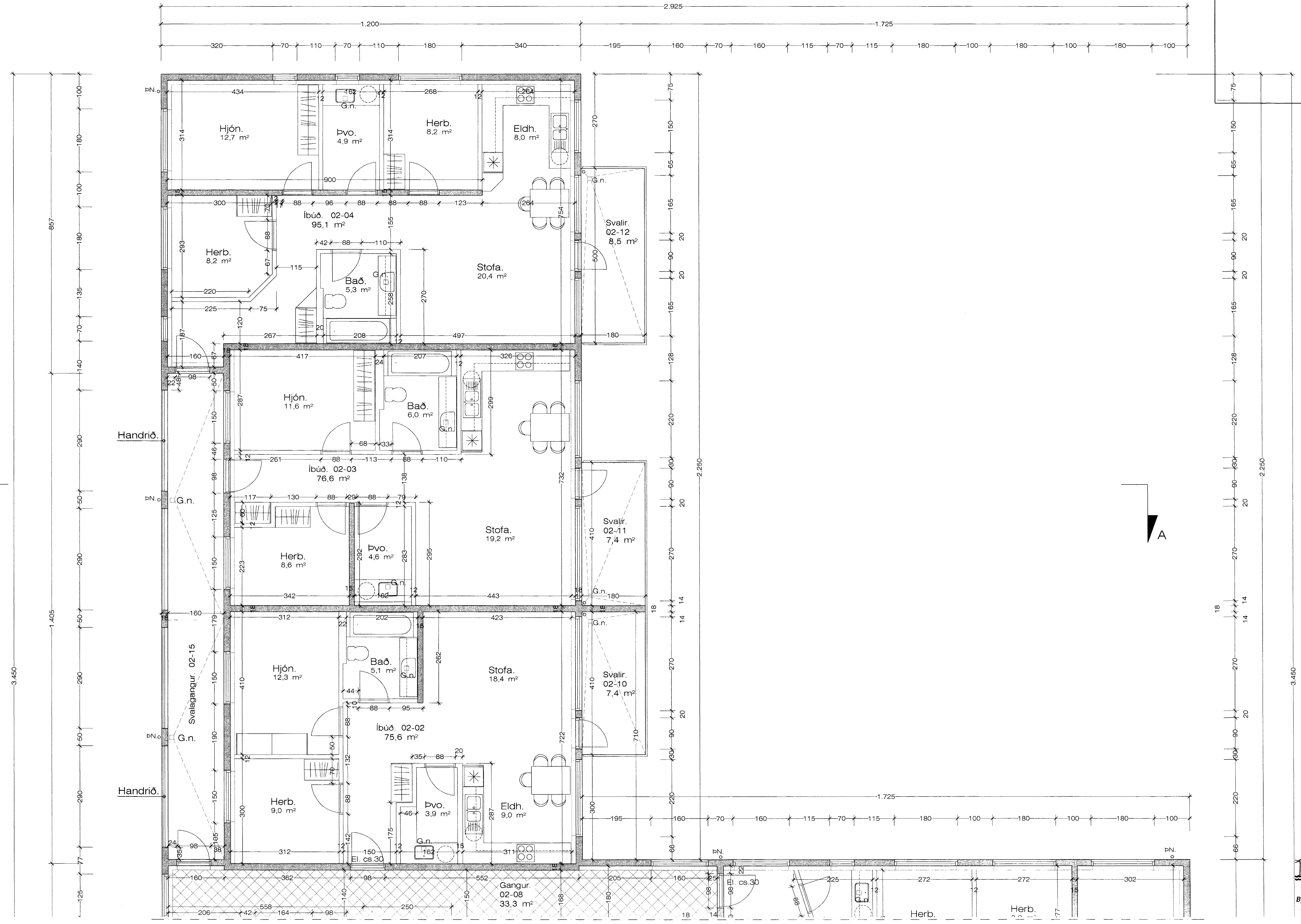
Grunnmynd. 2. - 3. hæð. B 1:50
