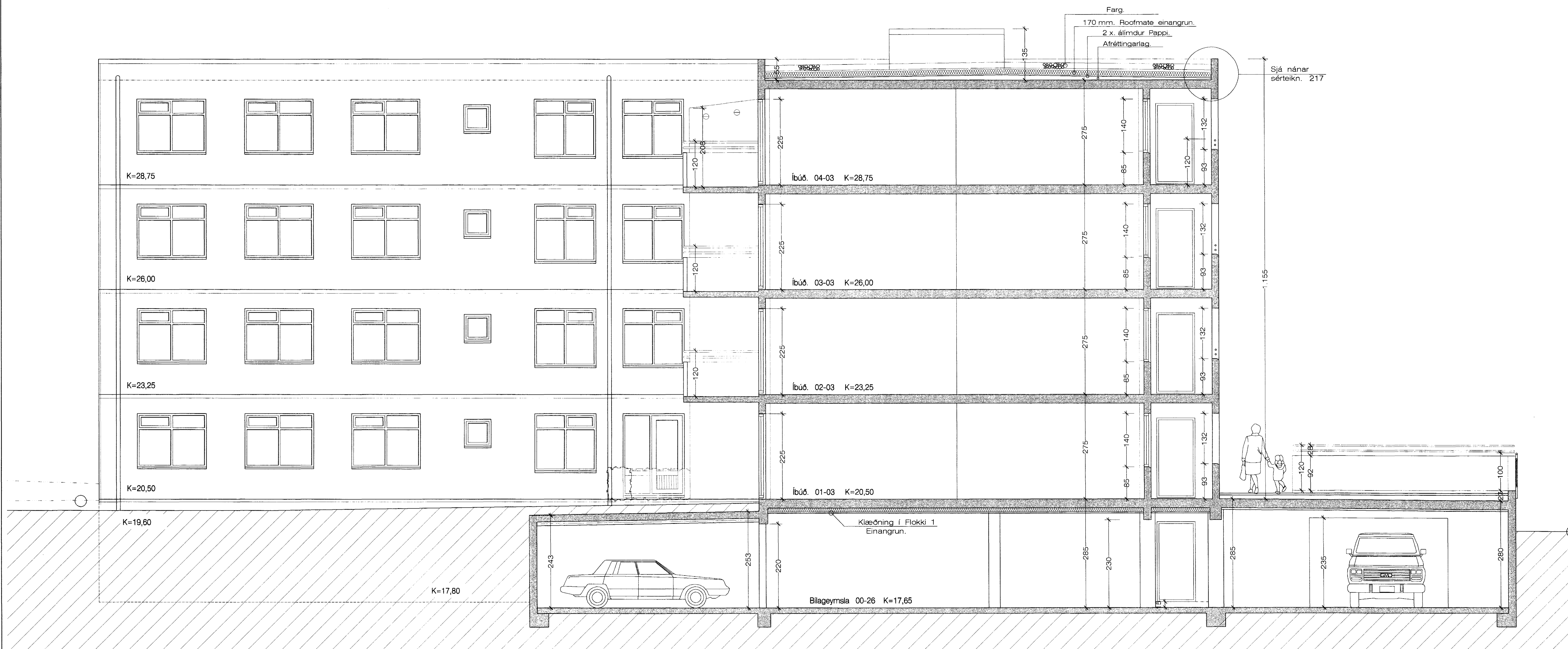
Sneiðing. A - A 1:50
