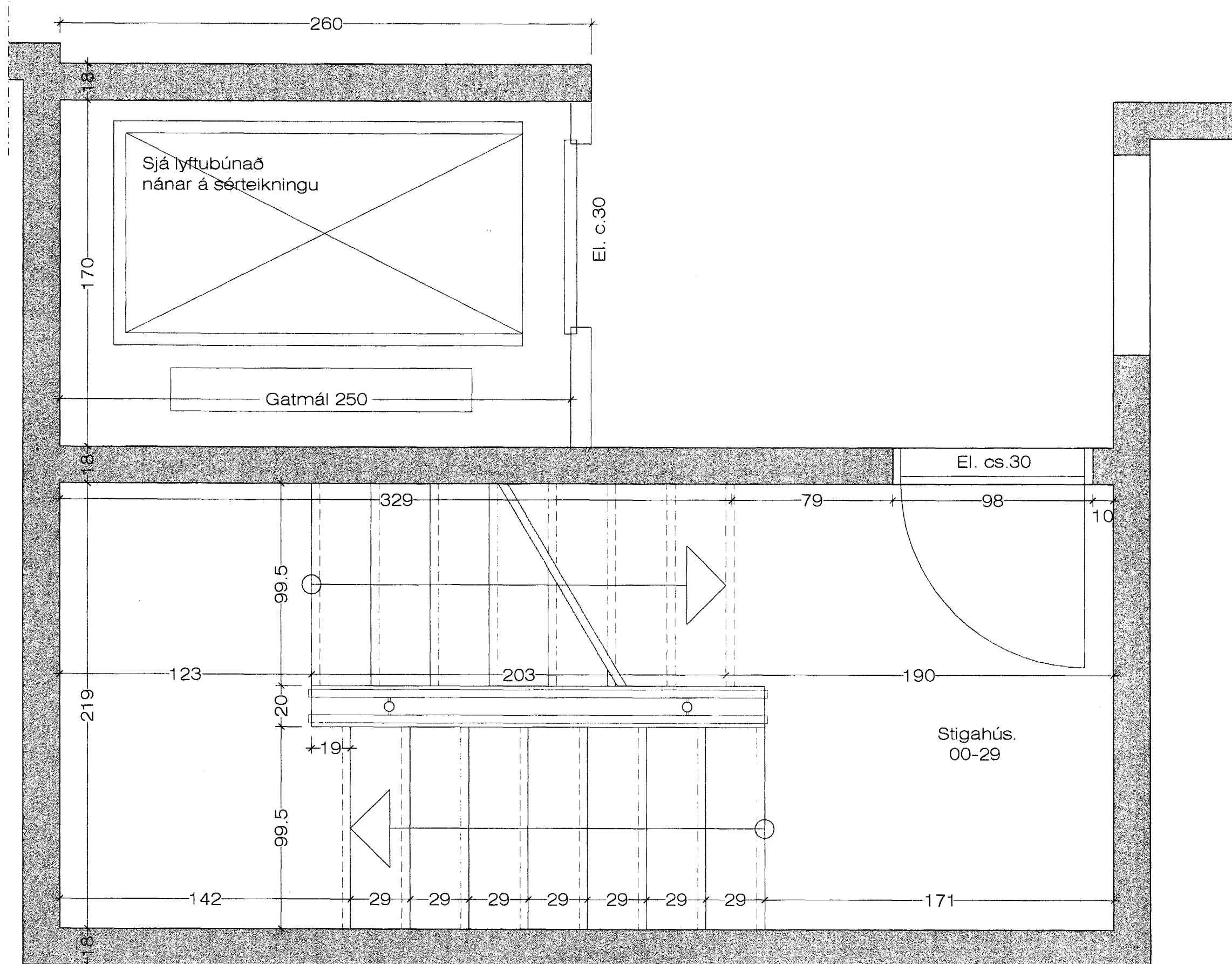
Grunmynd stíghús kjallara 1:20
