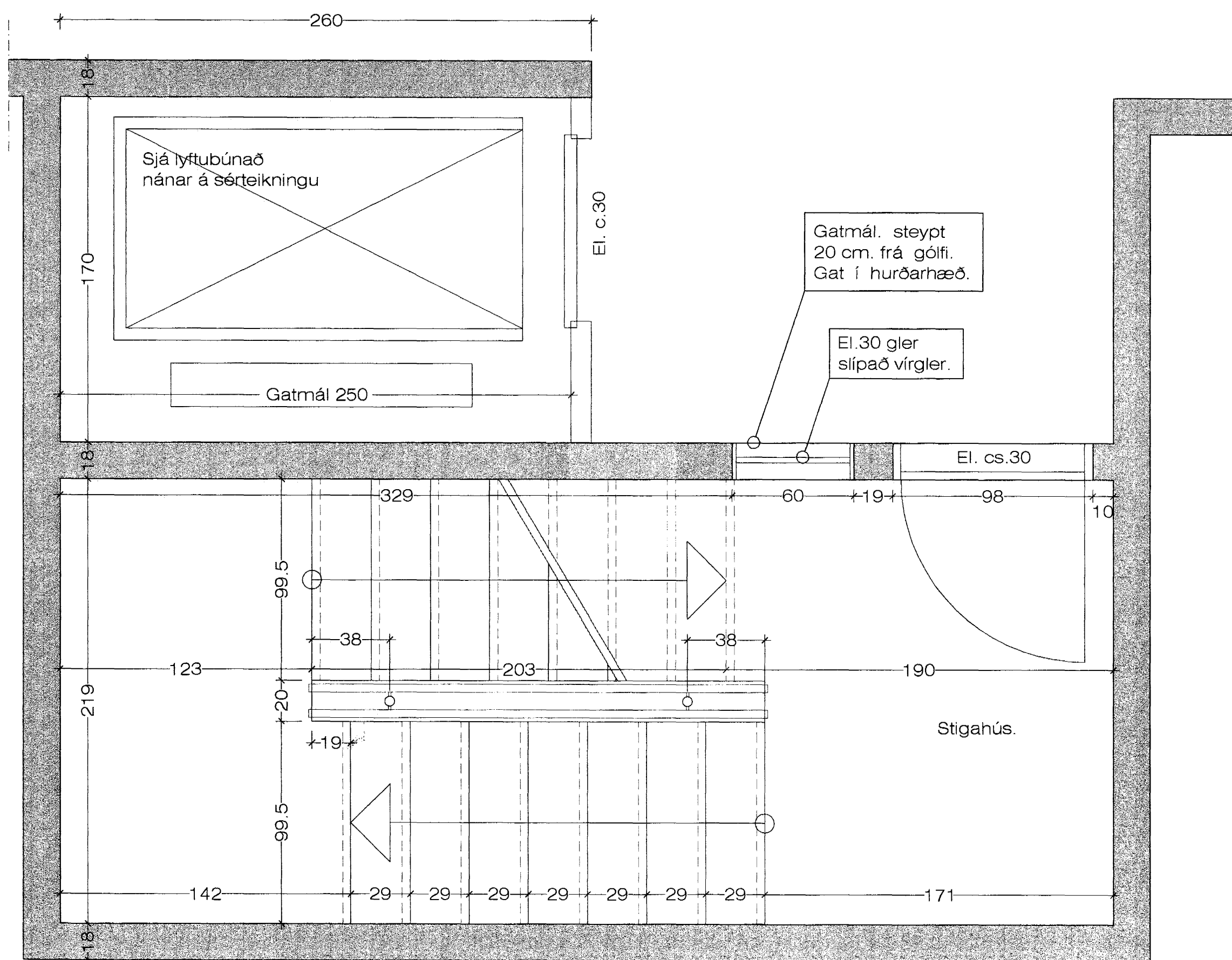
Grunmynd stíghús 1-4 hæð 1:20
