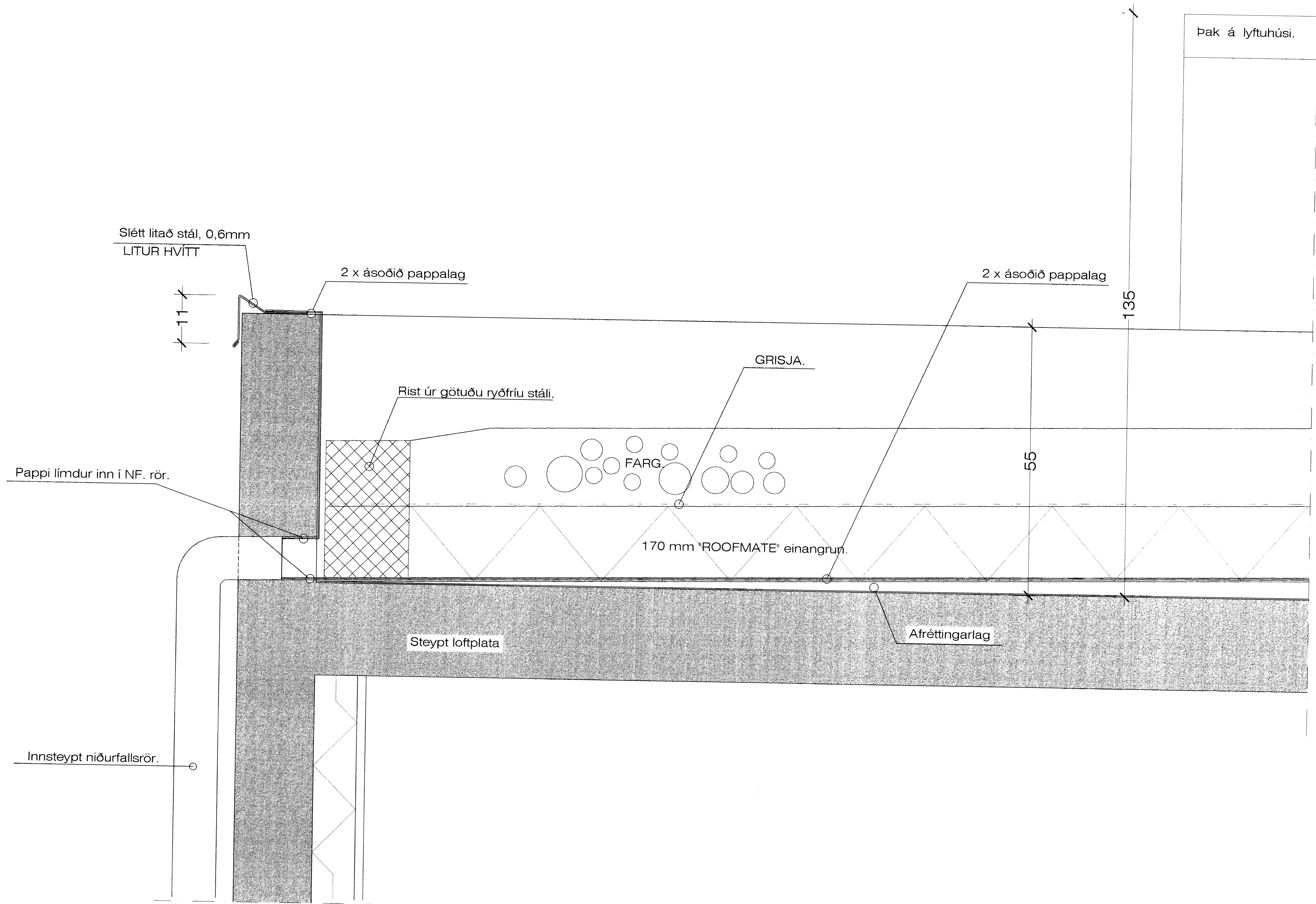
Frágangur á þakköntum. 1:5
