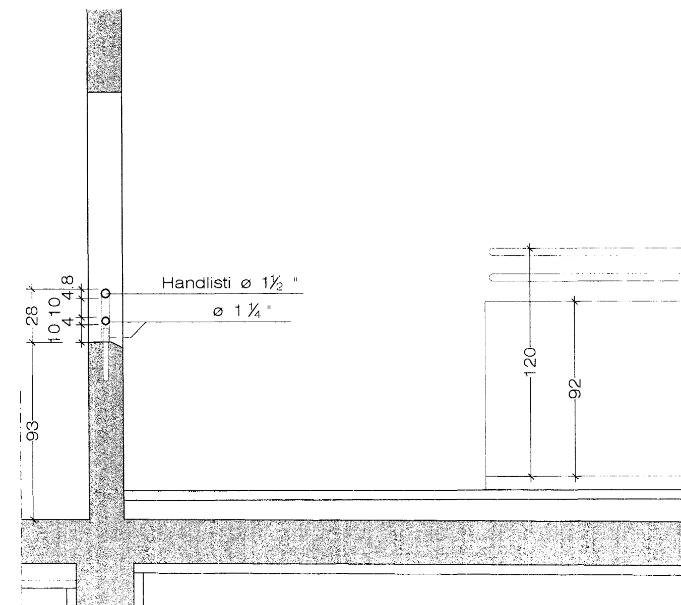
Handrið í götum á svalagangi. 1:20
