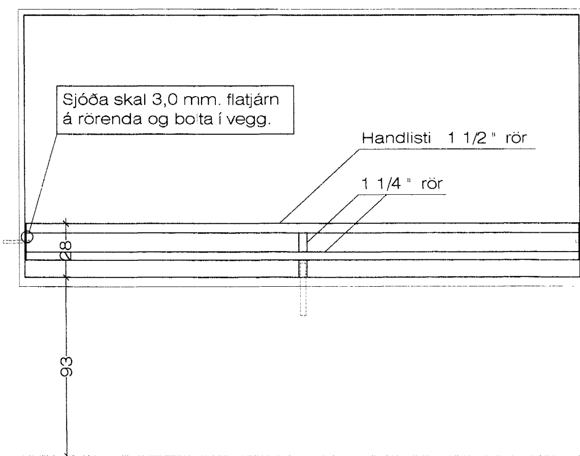
Handrið í götum á svalagangi. 1:20
