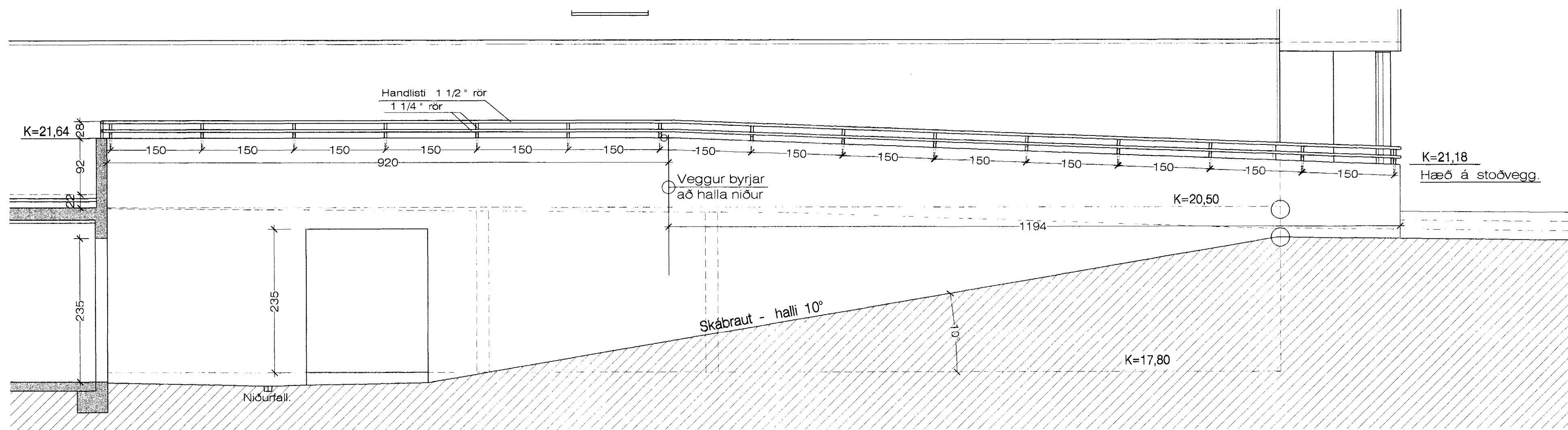
Hliðarmynd af handriði við niðurkeyrslu í bílahús. Við húshliðina. 1:50
