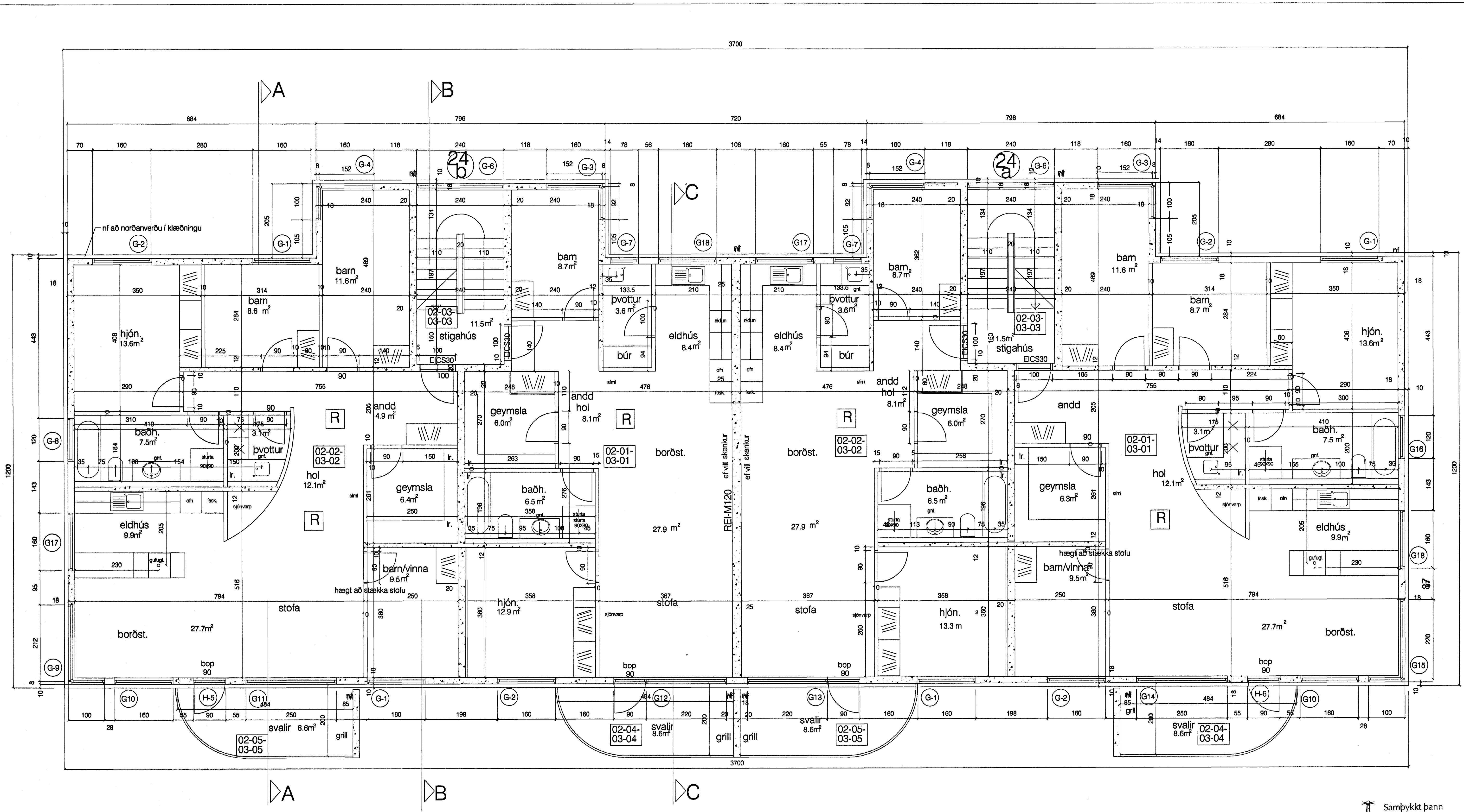
grunnmynd 2-3. hæð
