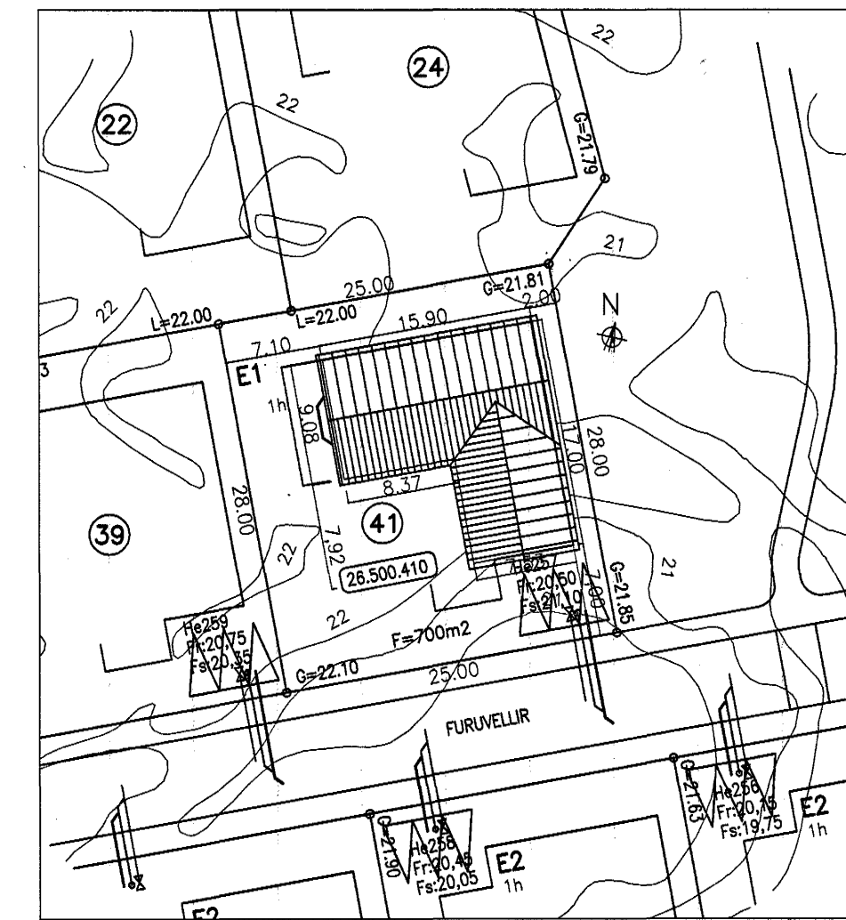
AFSTÖÐUMYND 1:500
