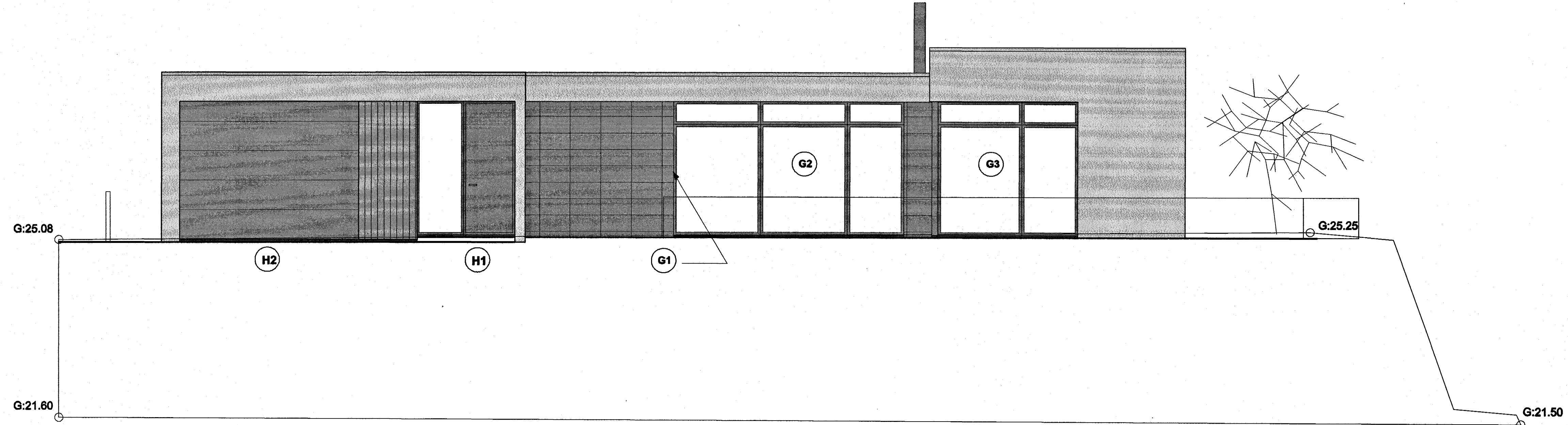
ÚTLIT SUÐVESTUR
