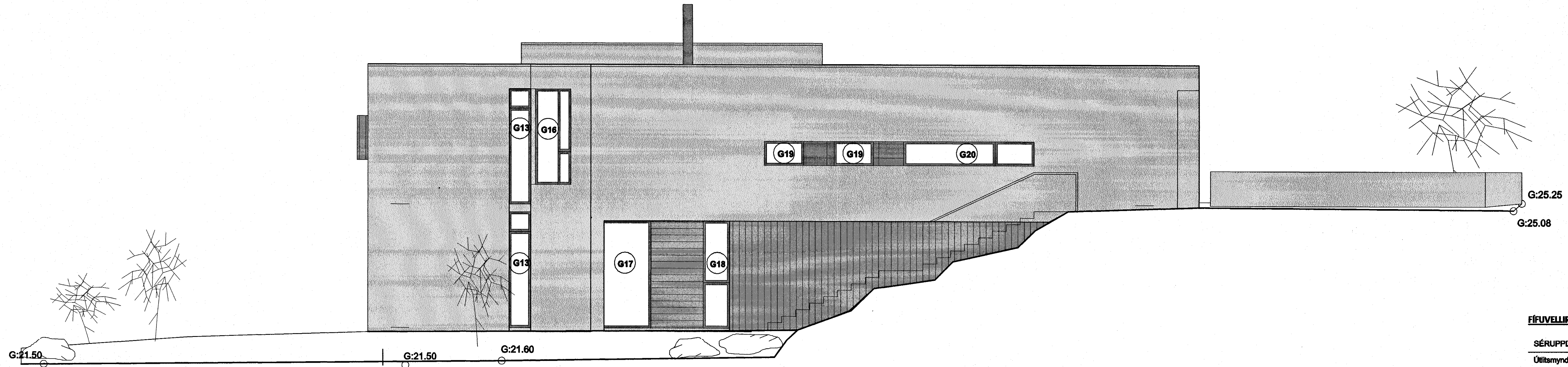
ÚTLIT NORÐVESTUR
