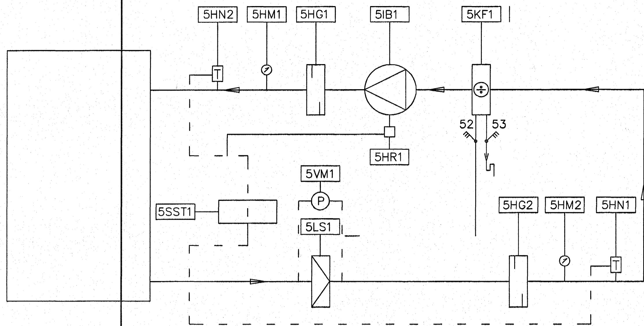
D KÆLIKERFI 5 - KÆLIKERFI - Netþjónn. 1H 501/506 KERFISMYND
