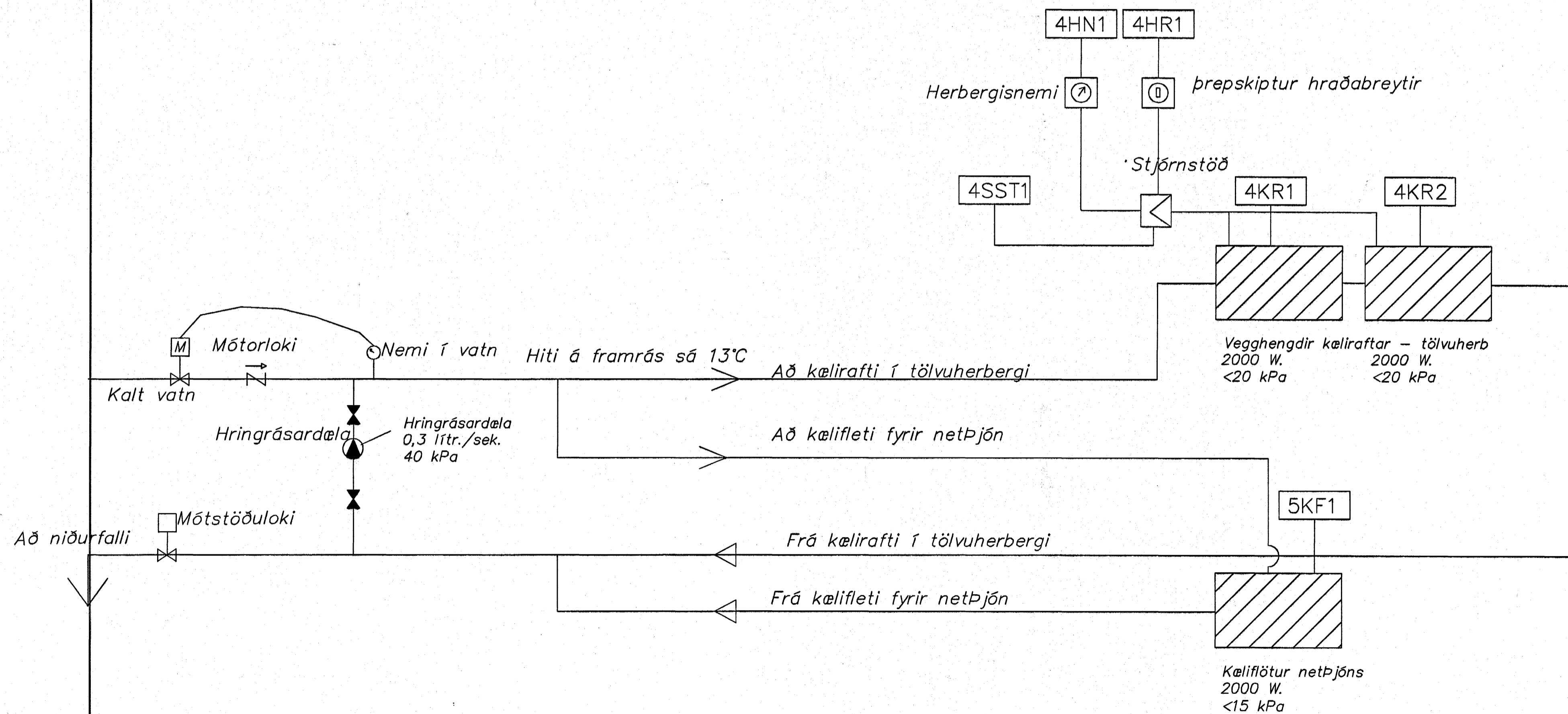
E KÆLIKERFI 4 - KÆLIKERFI - TÖLVUHERB. 1H 501/506 KERFISMYND
