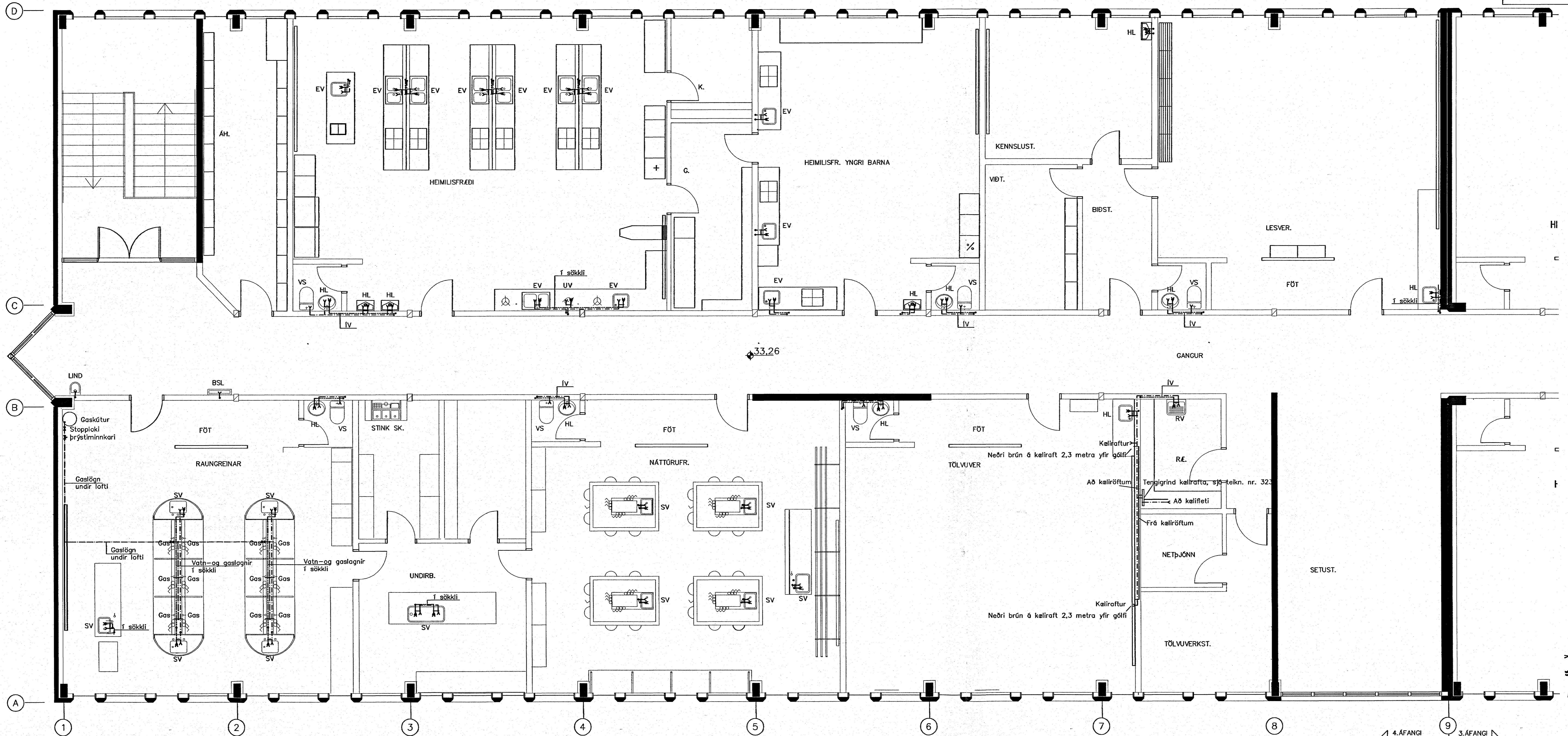
Grunnmynd 1. hæð 1 = 50 mm
