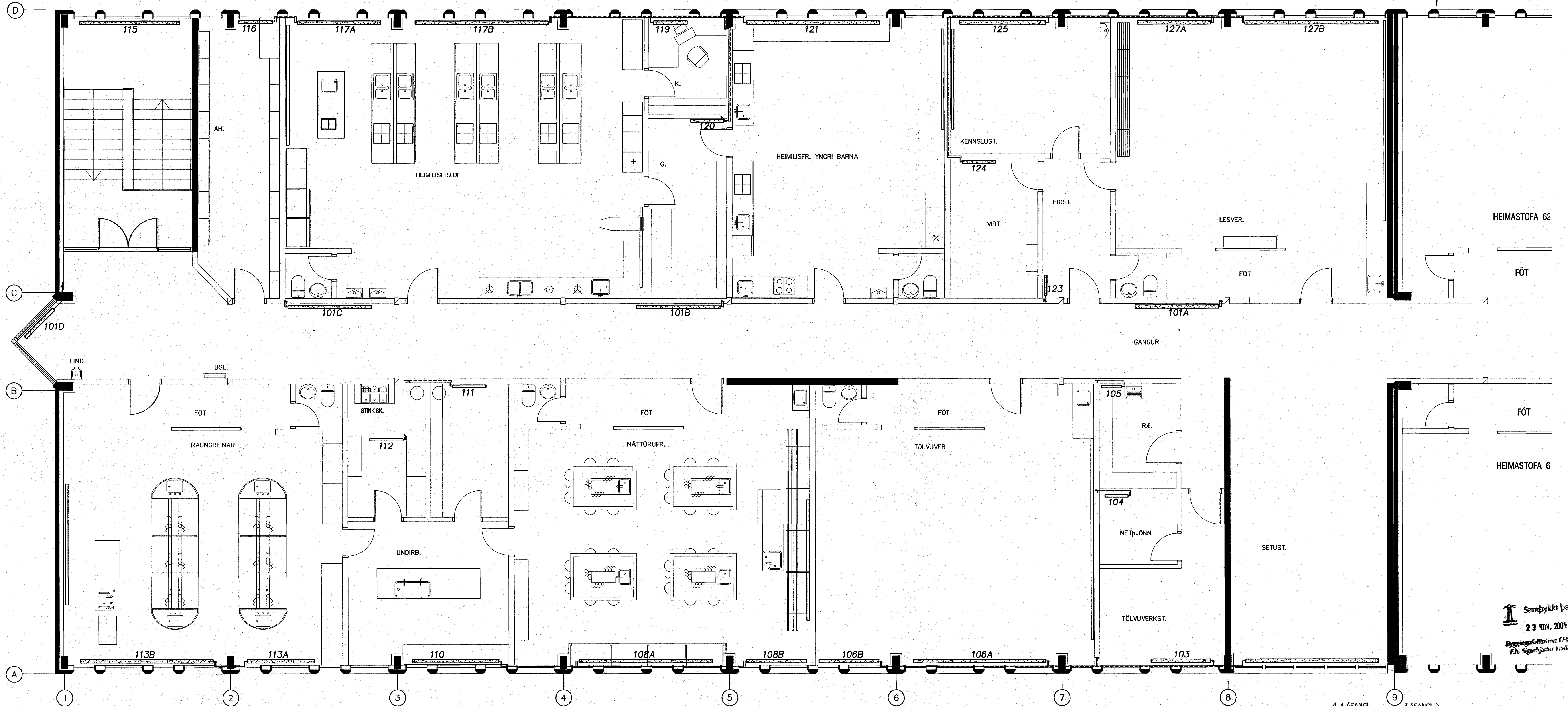
Grunnmynd 1.hæð 1 = 50 mm
