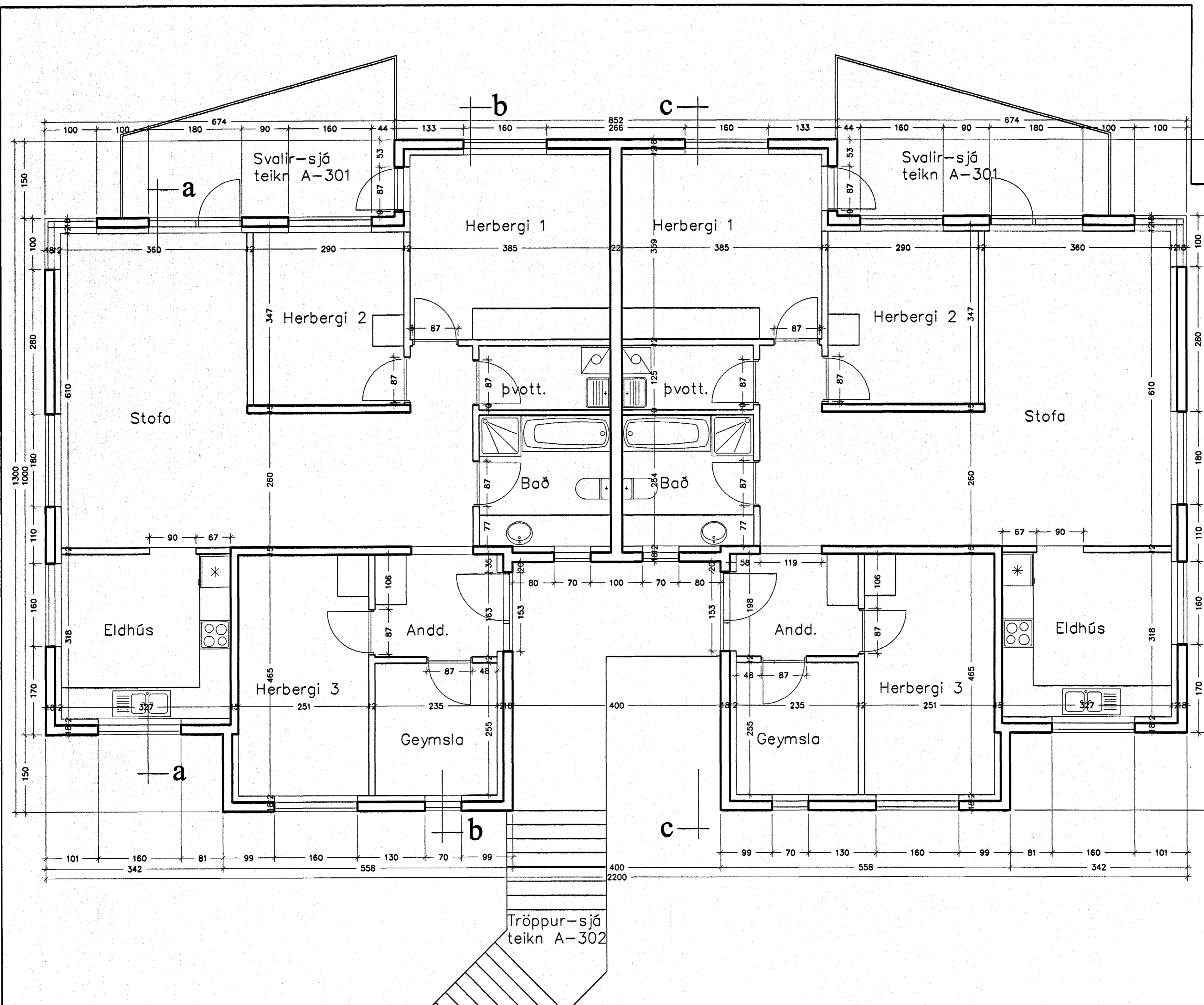
GRUNNMYND 1.HÆÐ 1:50
