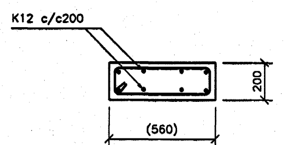
SÉRMYND 2 1:20
