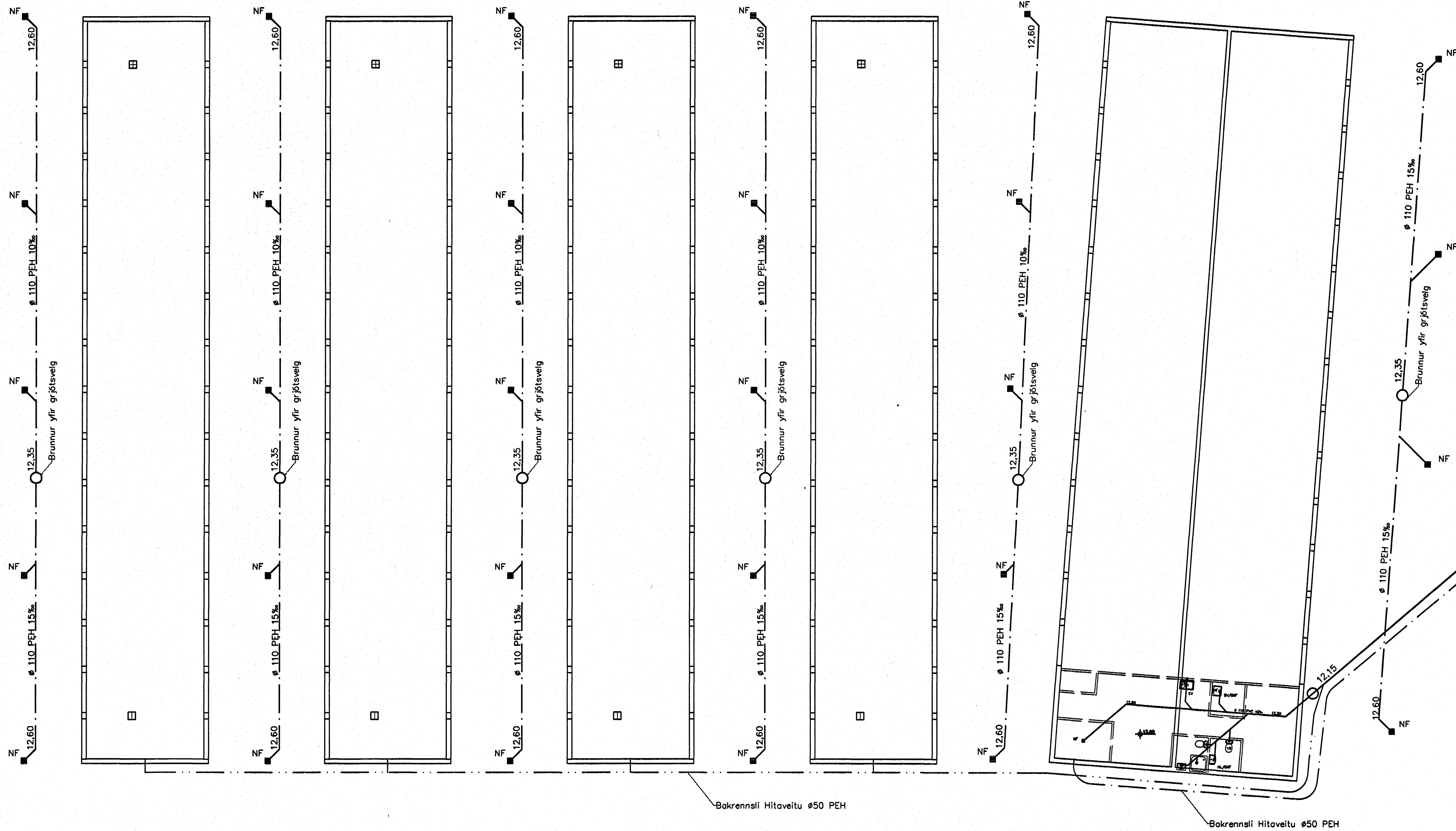
Fráveitulagnir, Grunnmynd, 1:125
