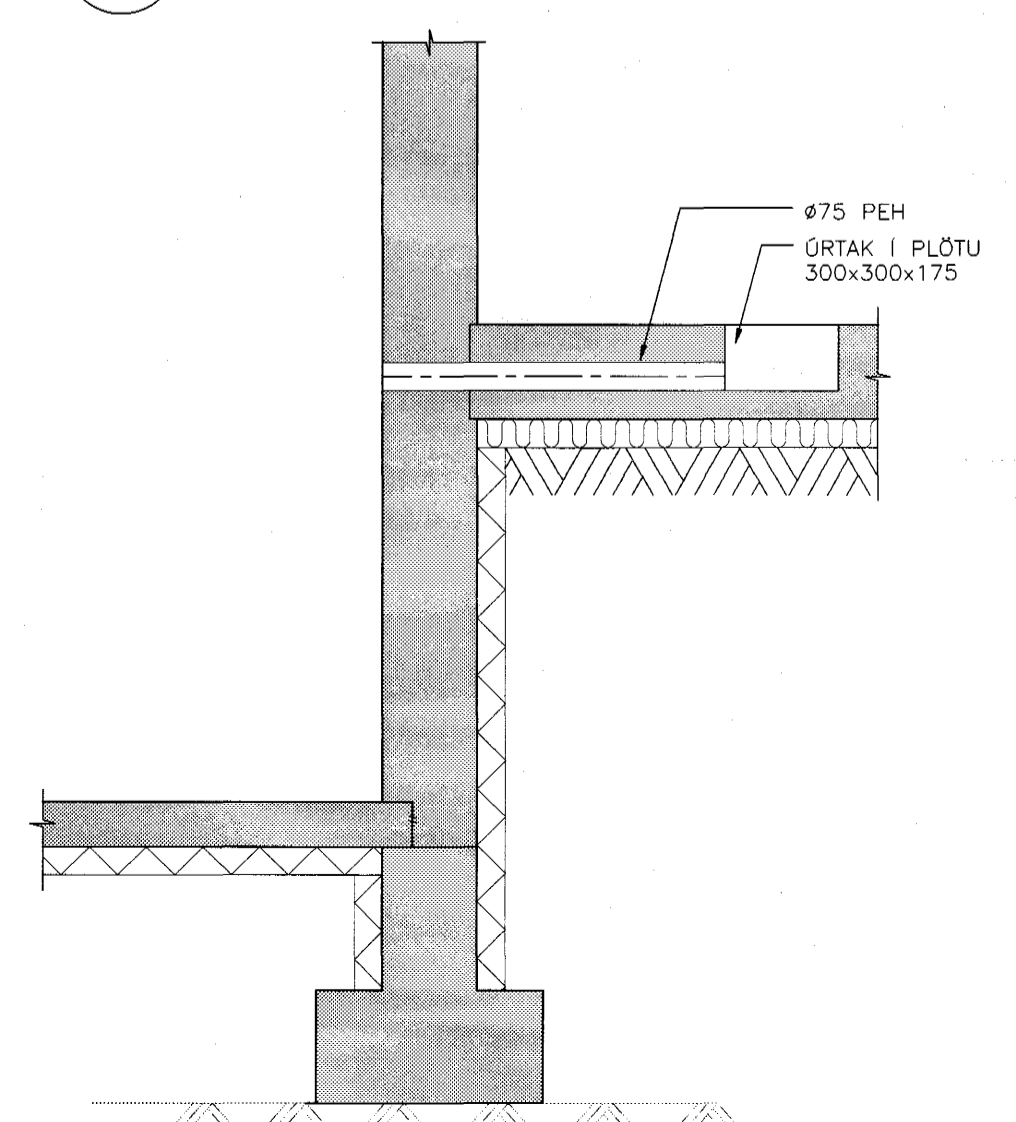
A SÉRMYND 1:20 FYRIR INNSTREYMI
