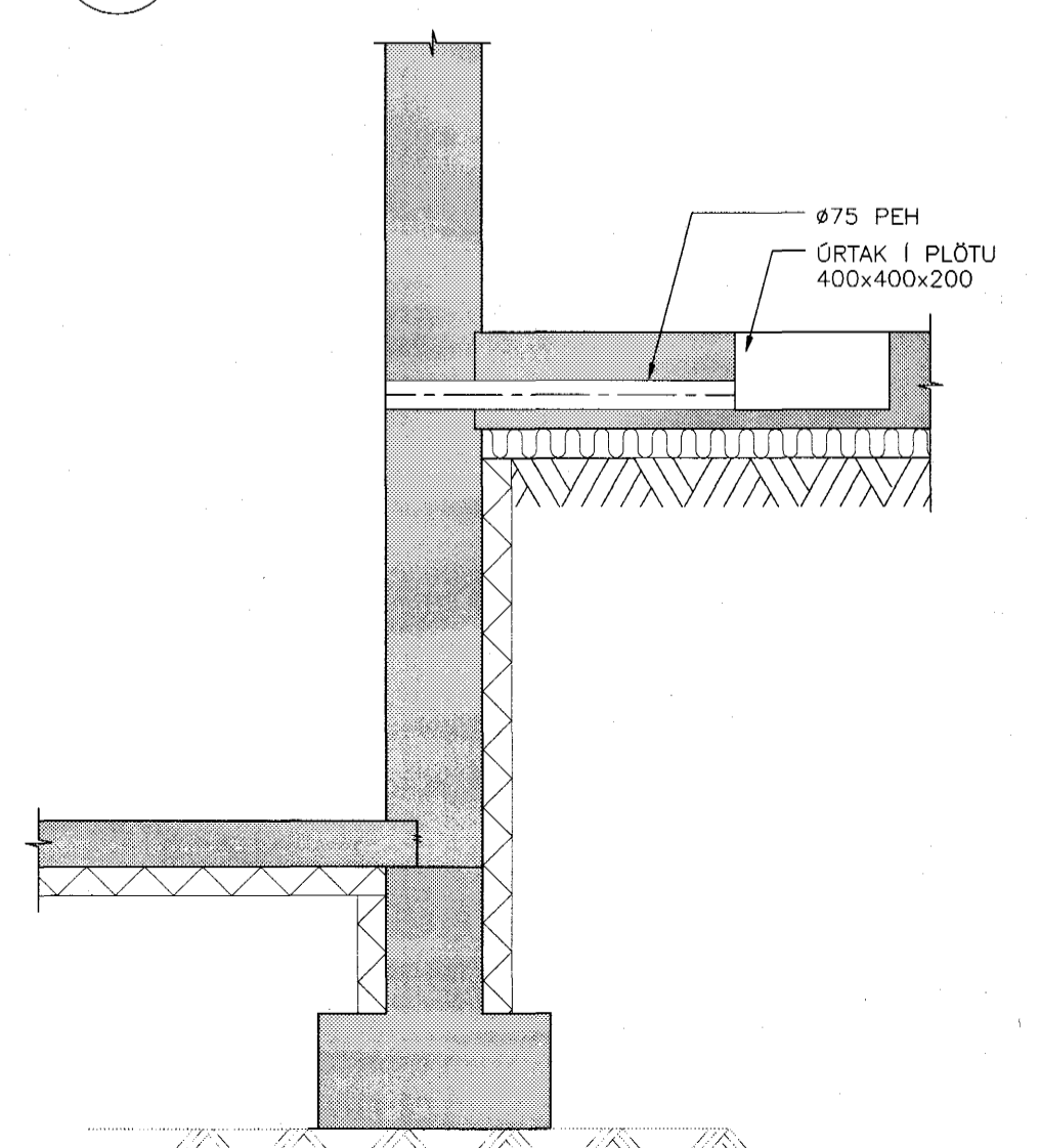
B SÉRMYND 1:20 FYRIR NIDURFALL
