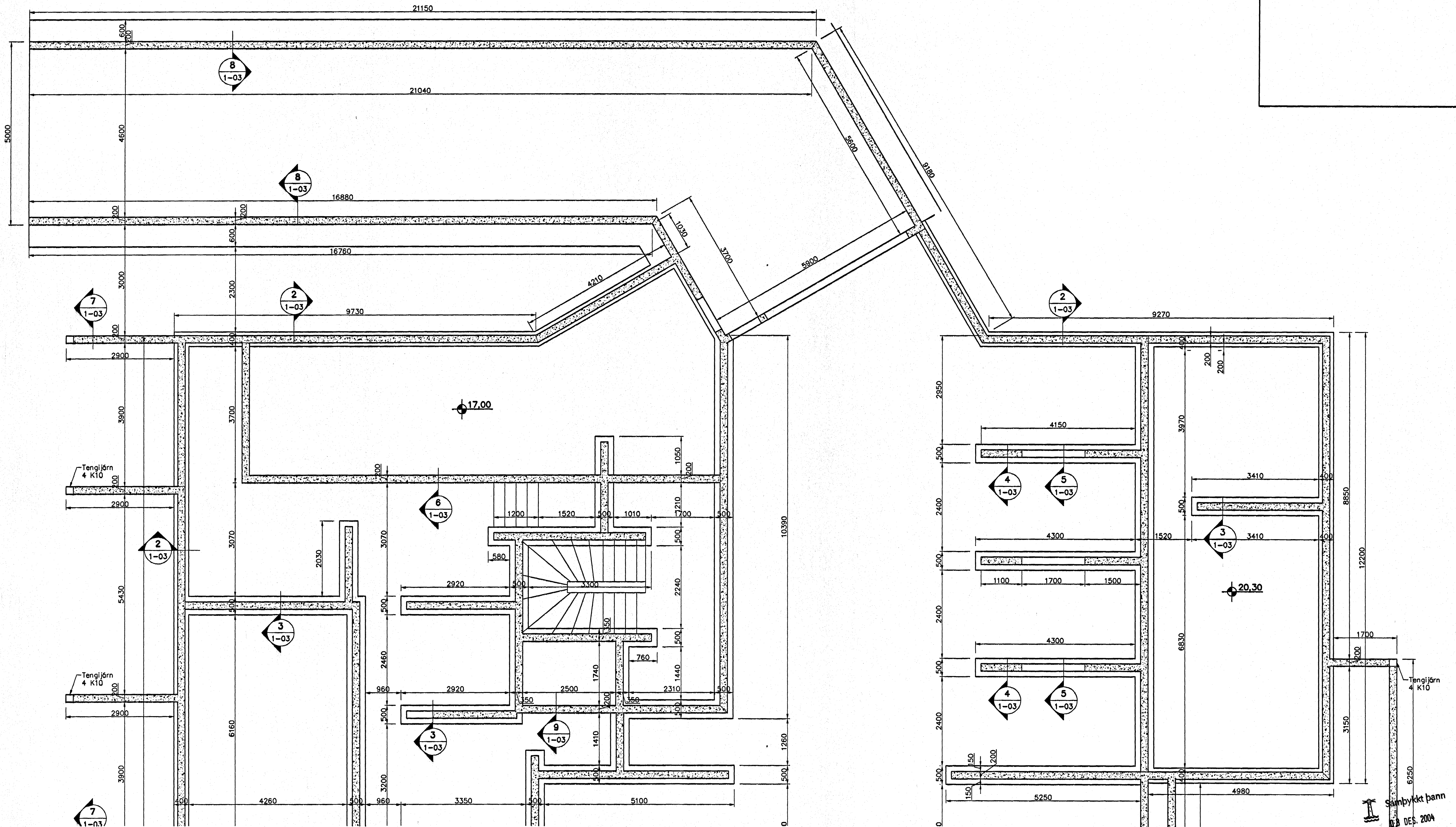
Undirstöður, Grunnmynd, 1:50
